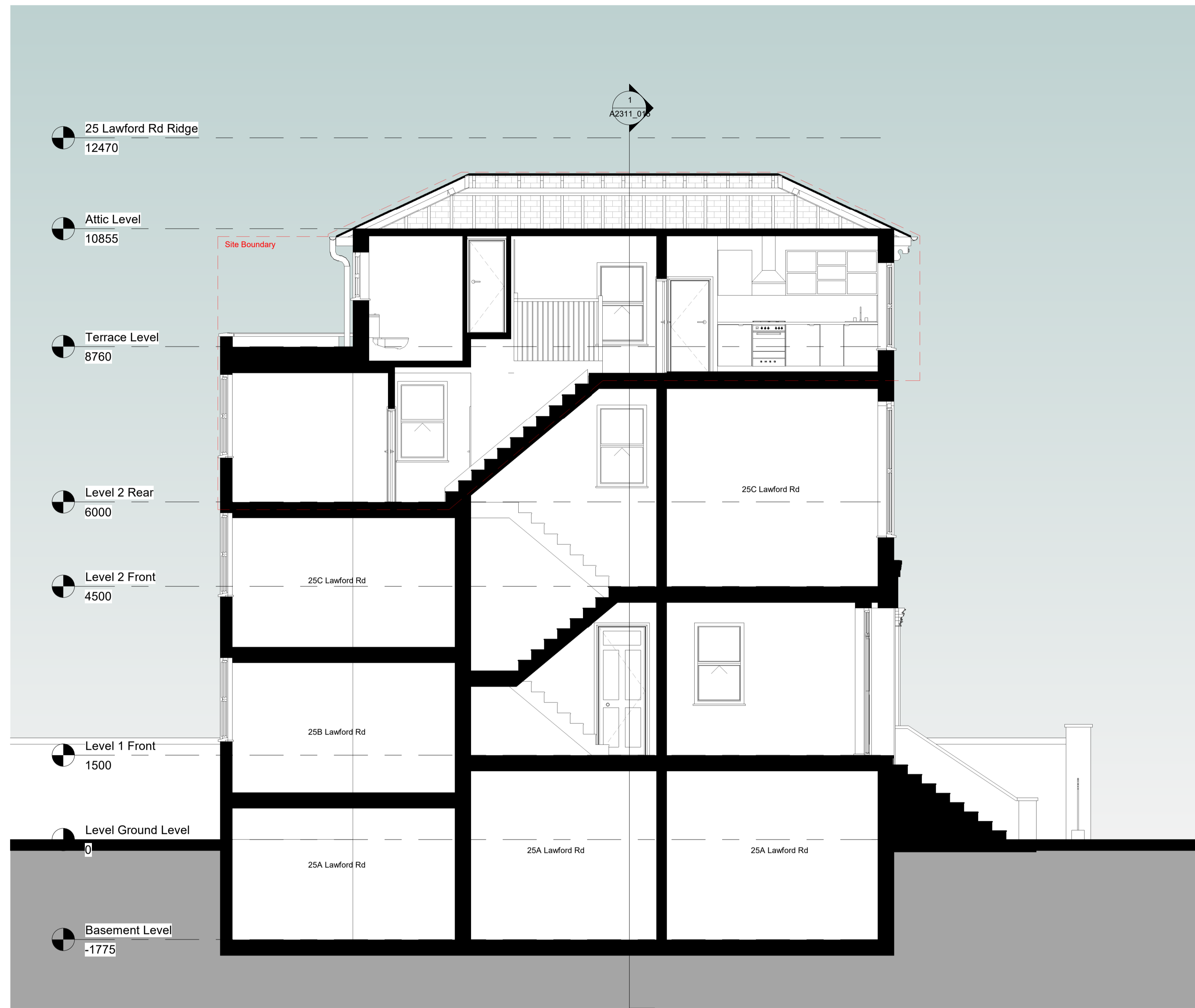
2 Existing Section B-B 1 : 50
