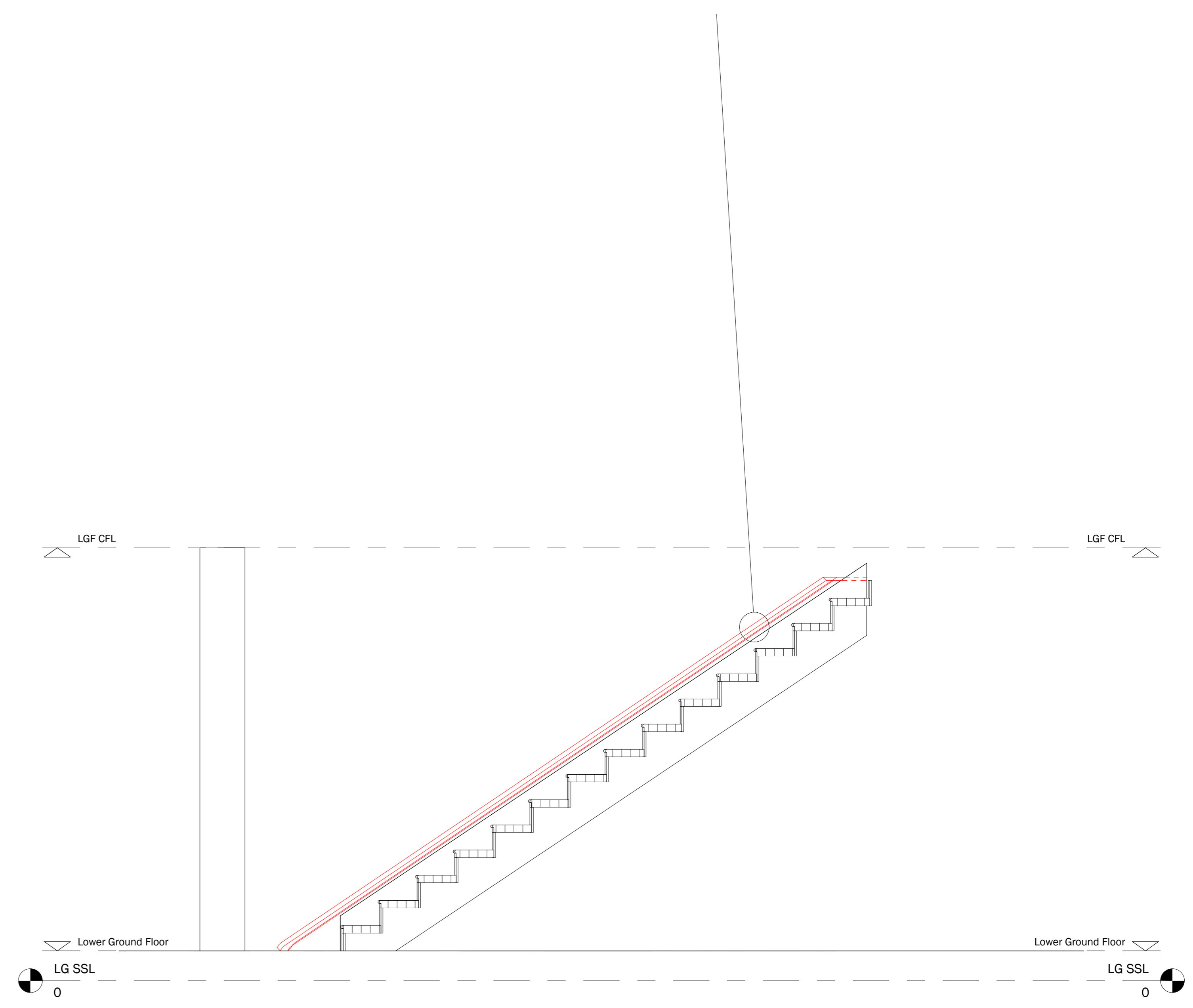
2 Section 10 1 : 20
