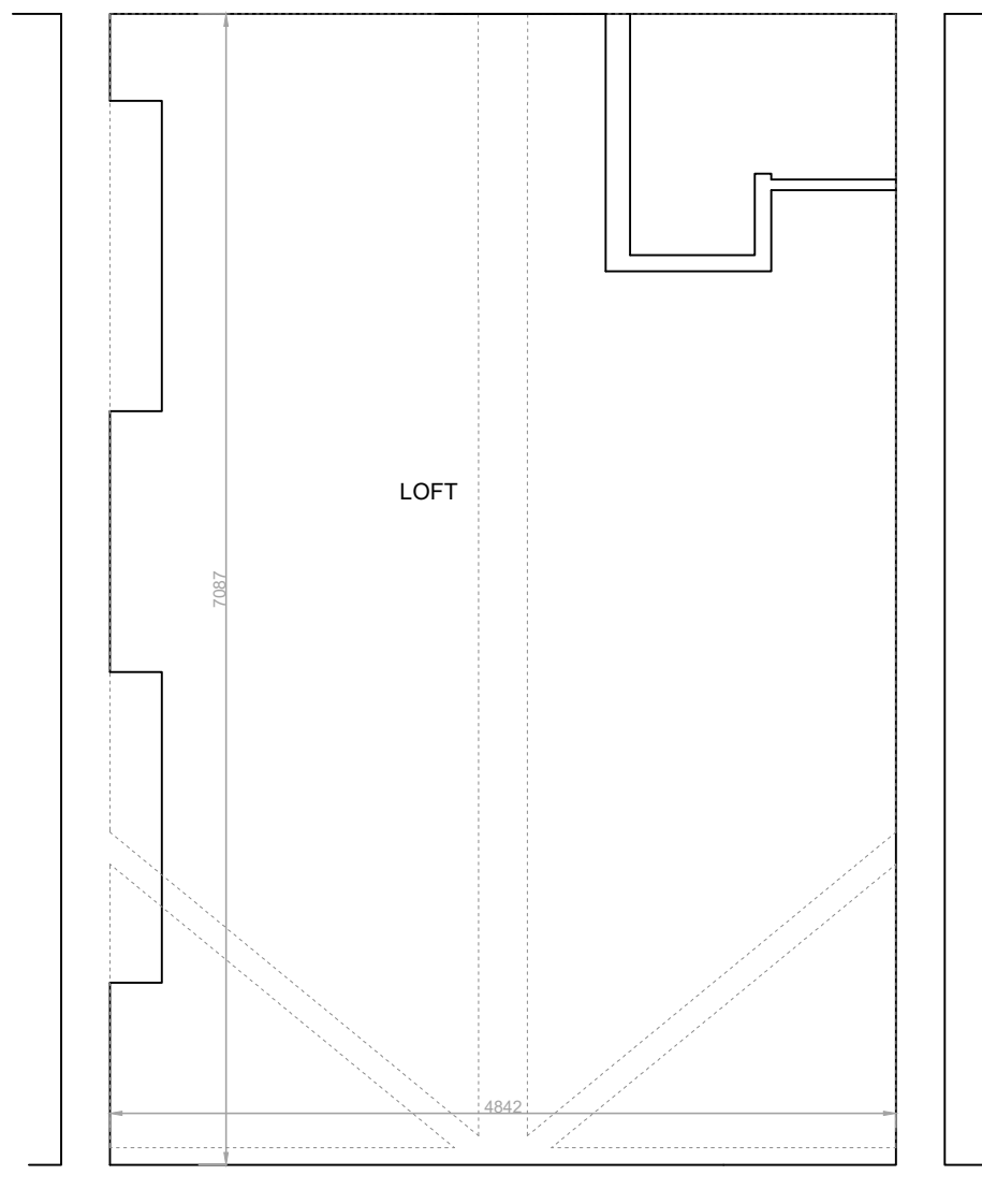
LOFT PLAN
