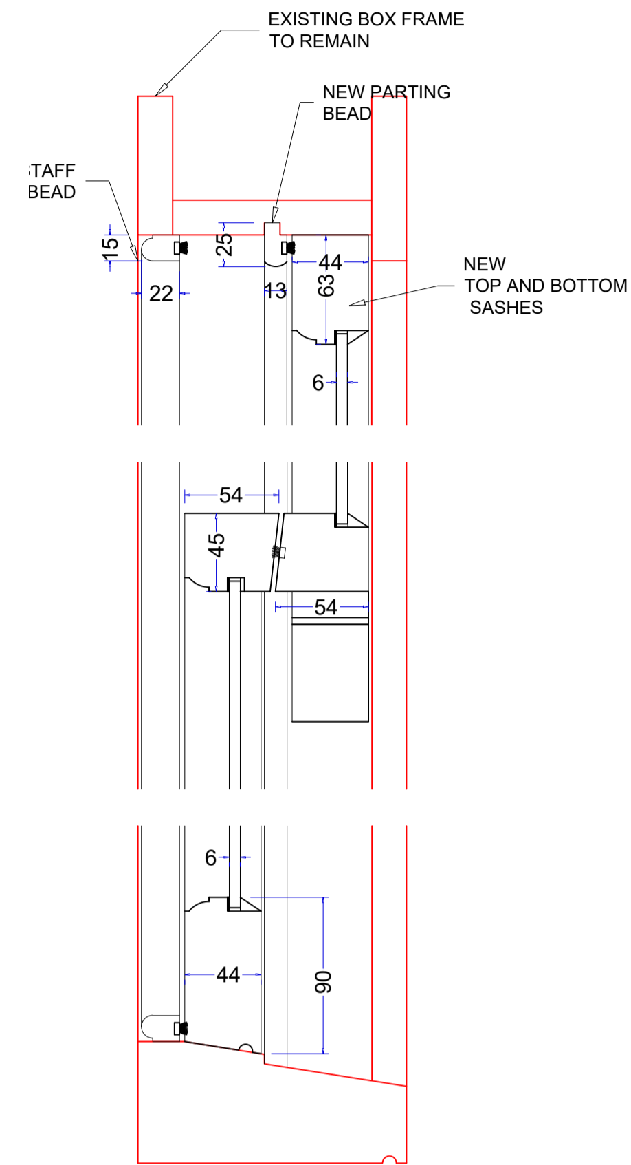
HEIGHT SECTION Scale: 1:3 @A1
