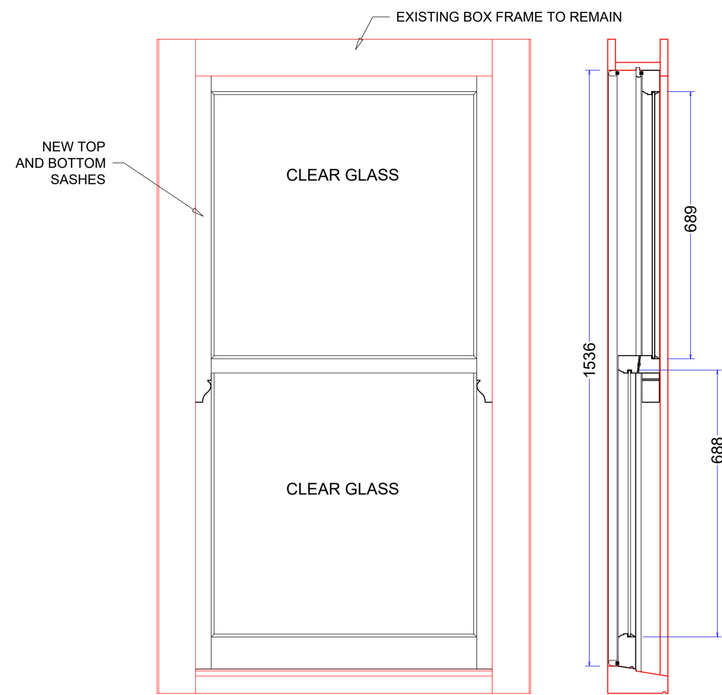
ELEVATION Scale: 1:2 @A1
