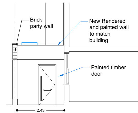
4_7a Front door elevation
