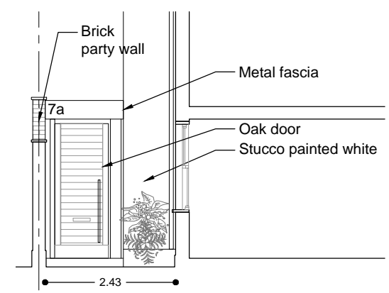
4_7a Front door elevation
