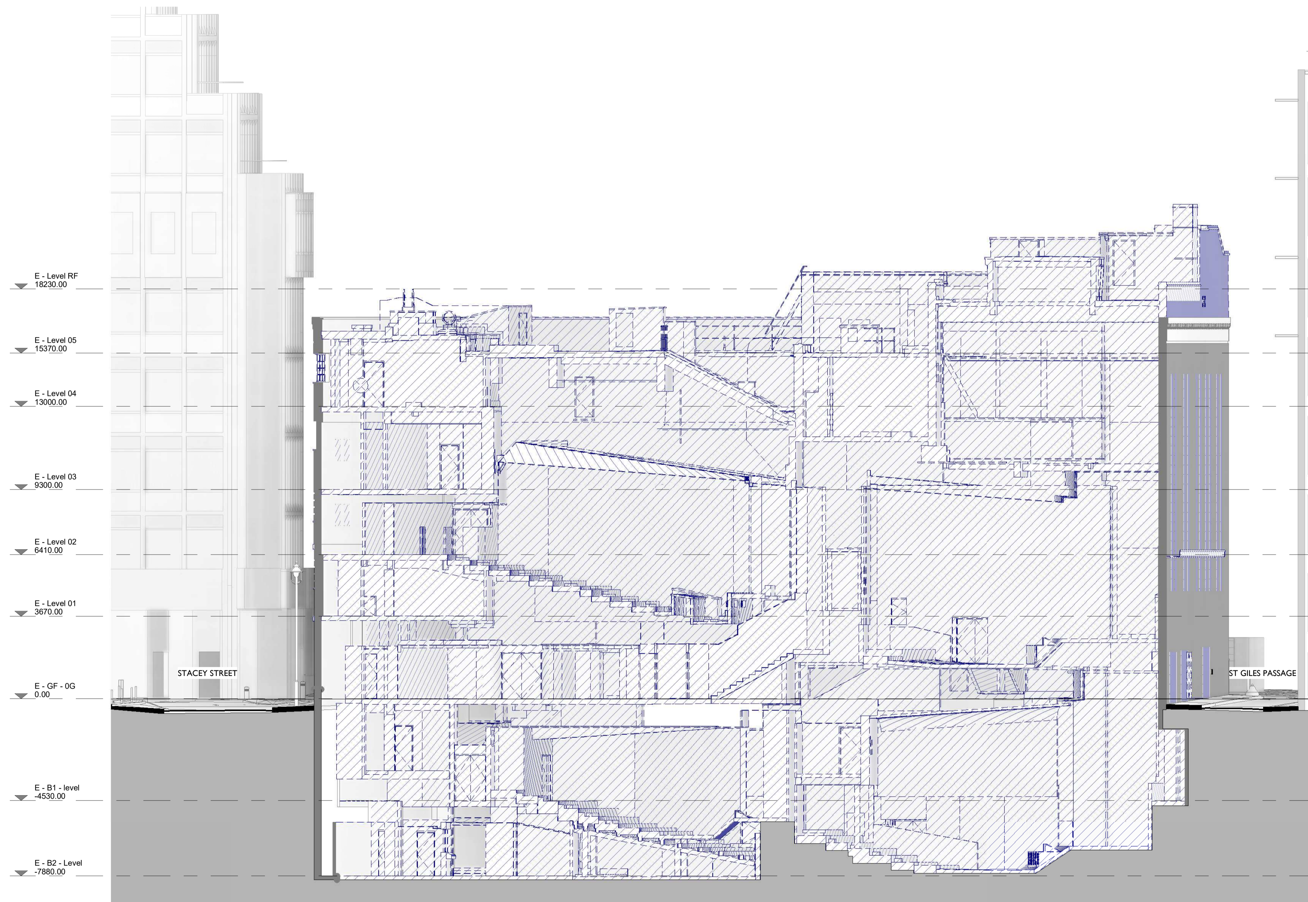
95-2001 - Section 1 1 : 100
