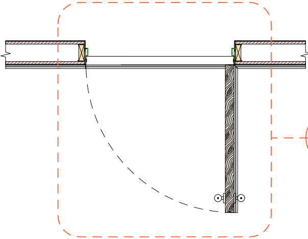
P Jib Door Plan 1:20
