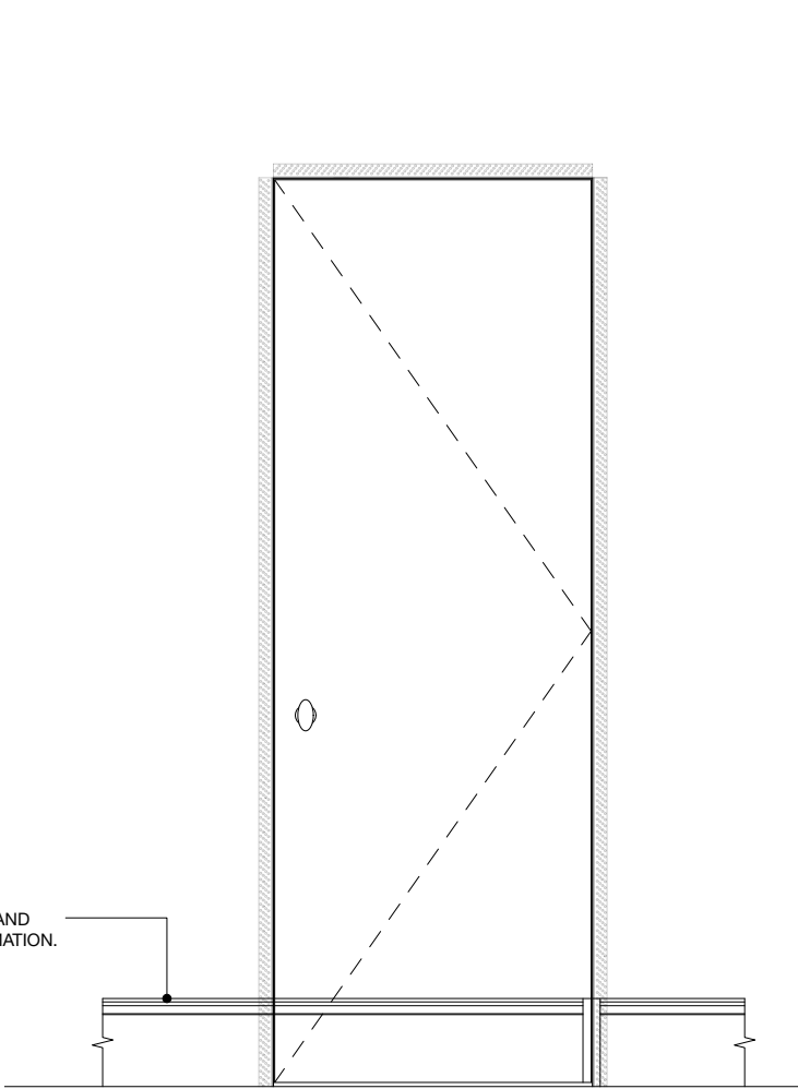
E Jib Door Elevation 1:20
