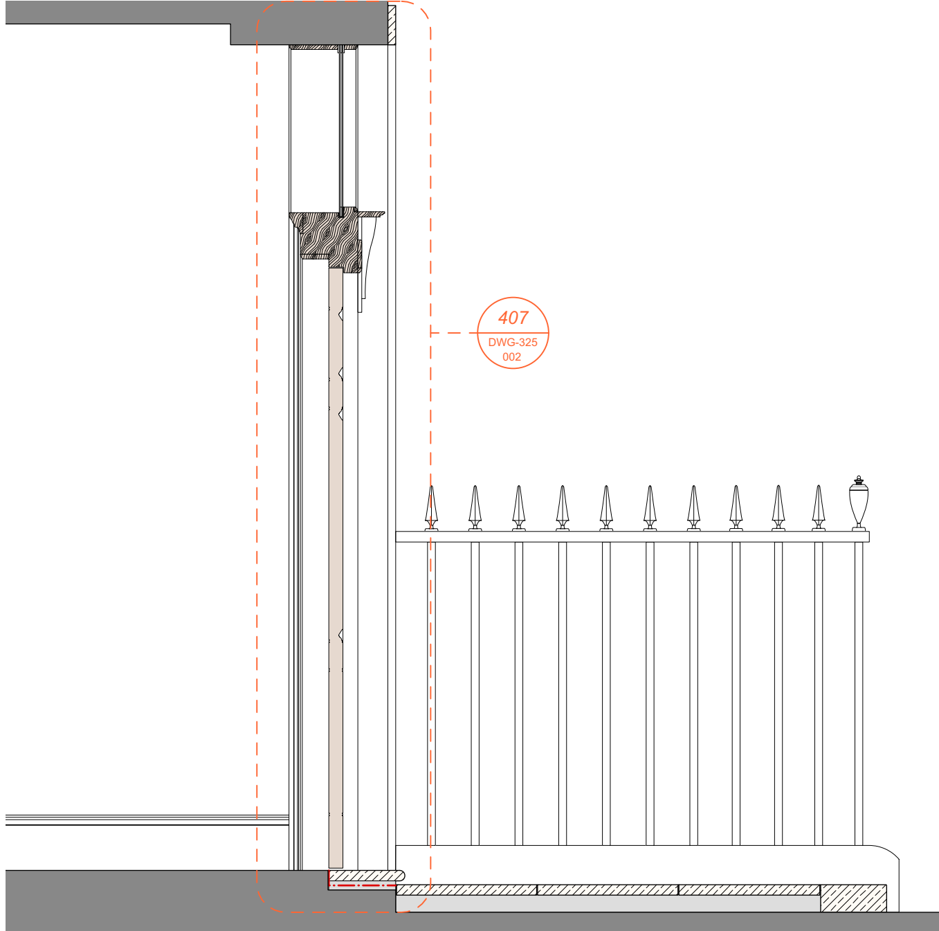
S Front Door Section 1:20
