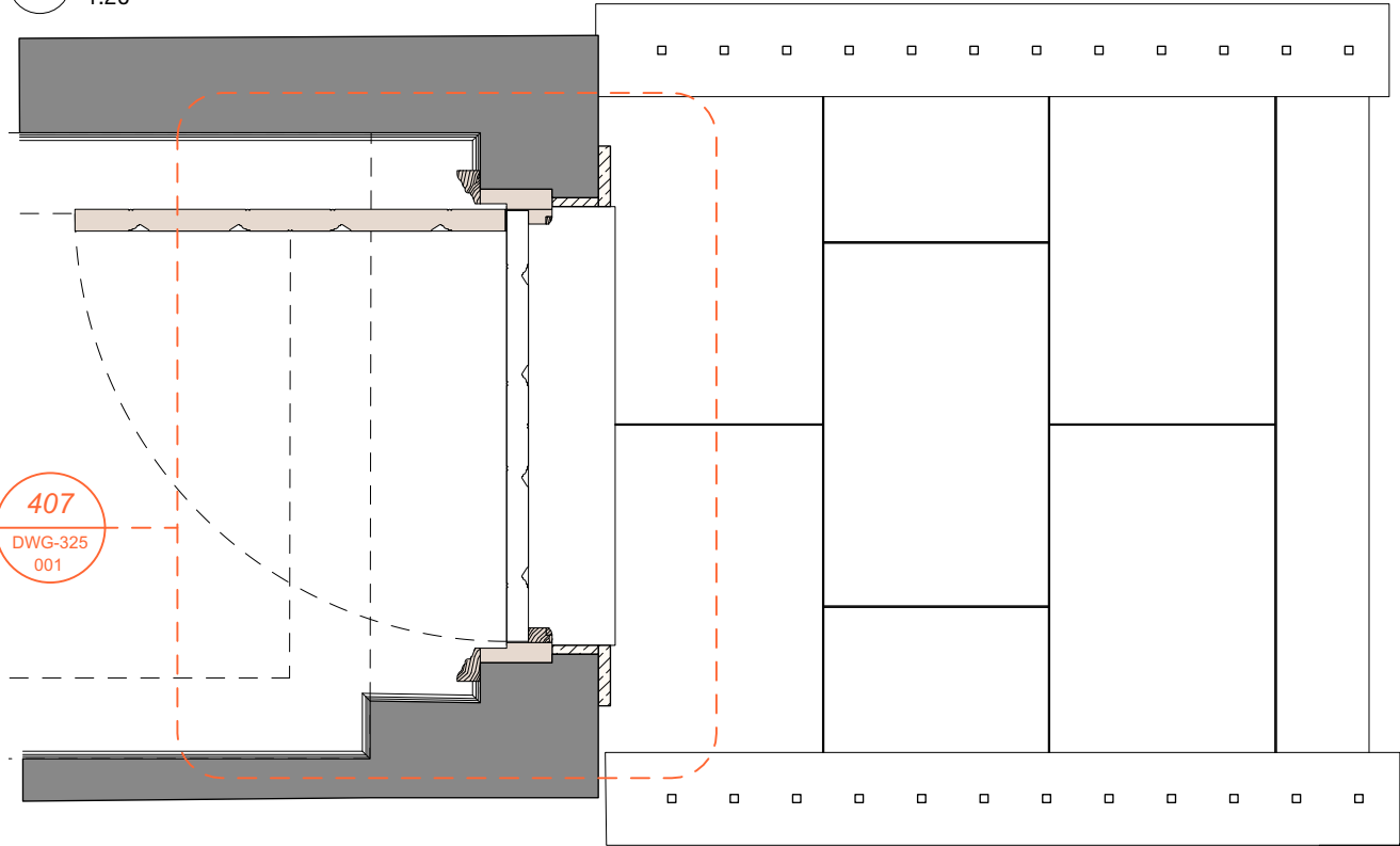
S Front Door Section 1:20
