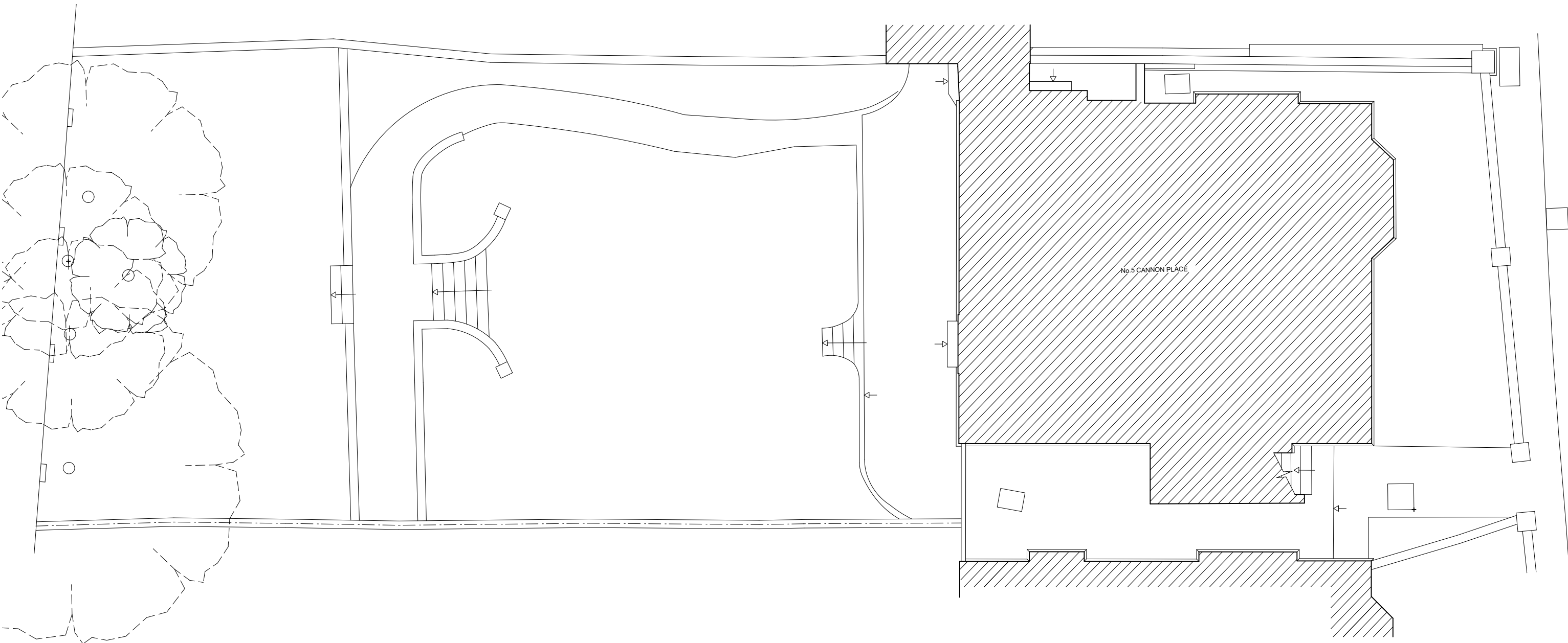
EXISTING SITE PLAN 1:100
