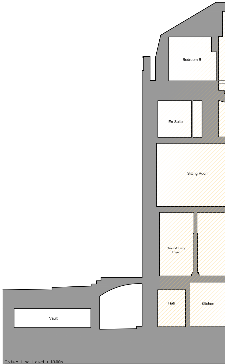
1 Existing Section B-B GHV 1:100 @ A3
