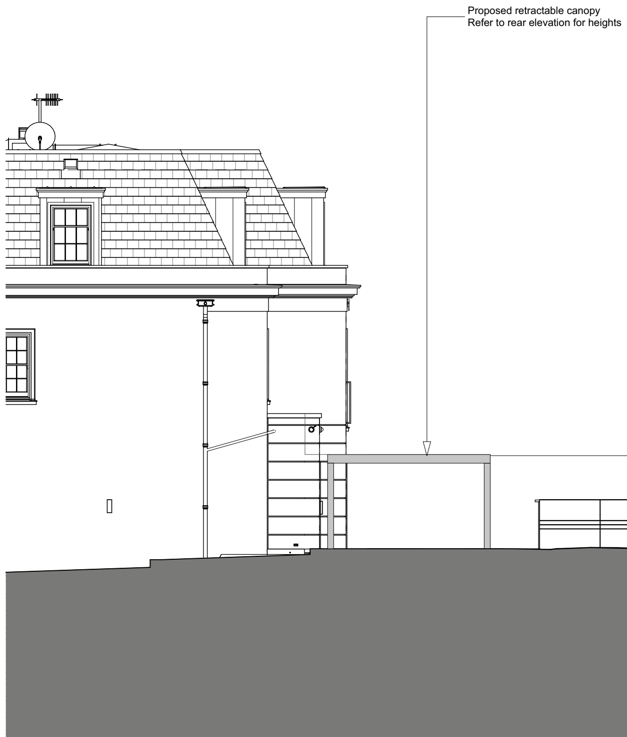
Part SE Elevation 1:100
