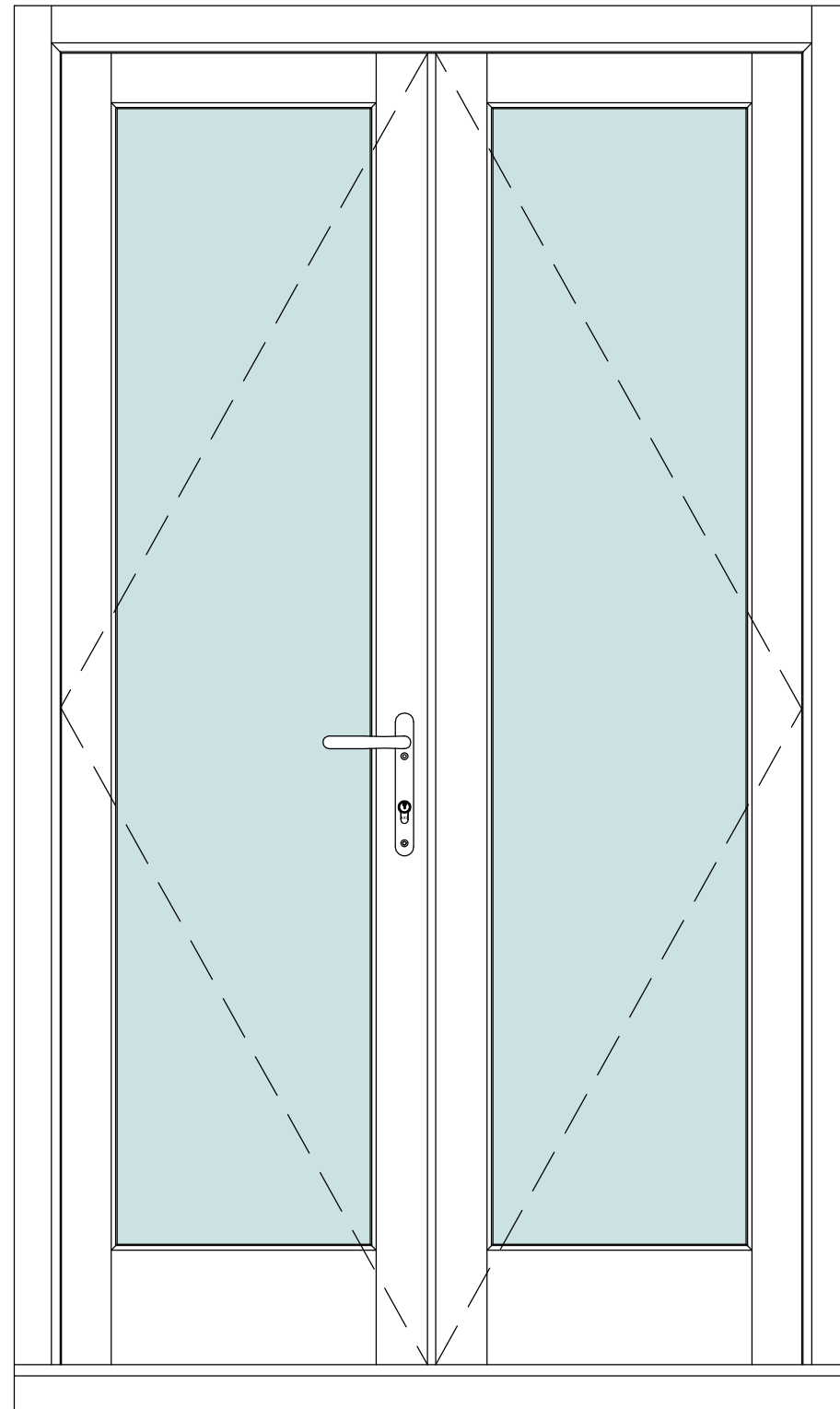
Door Overview Scale 1:10
