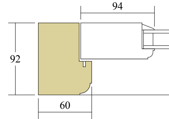
Jamb Section Scale 1:3
