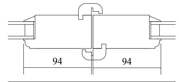
Door Rebate Section Scale 1:3
