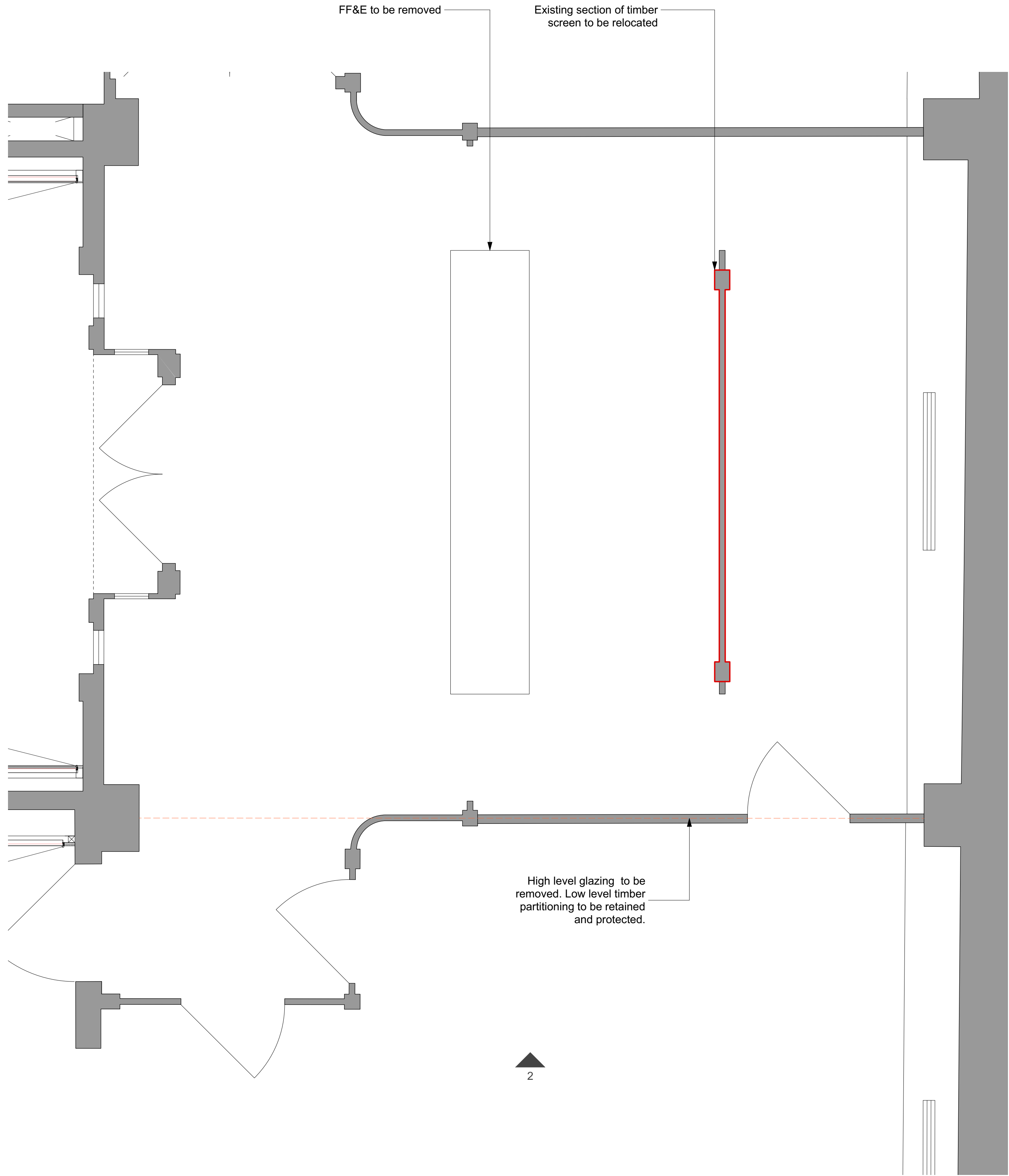
1 Existing Screen Plan Scale: 1:20
