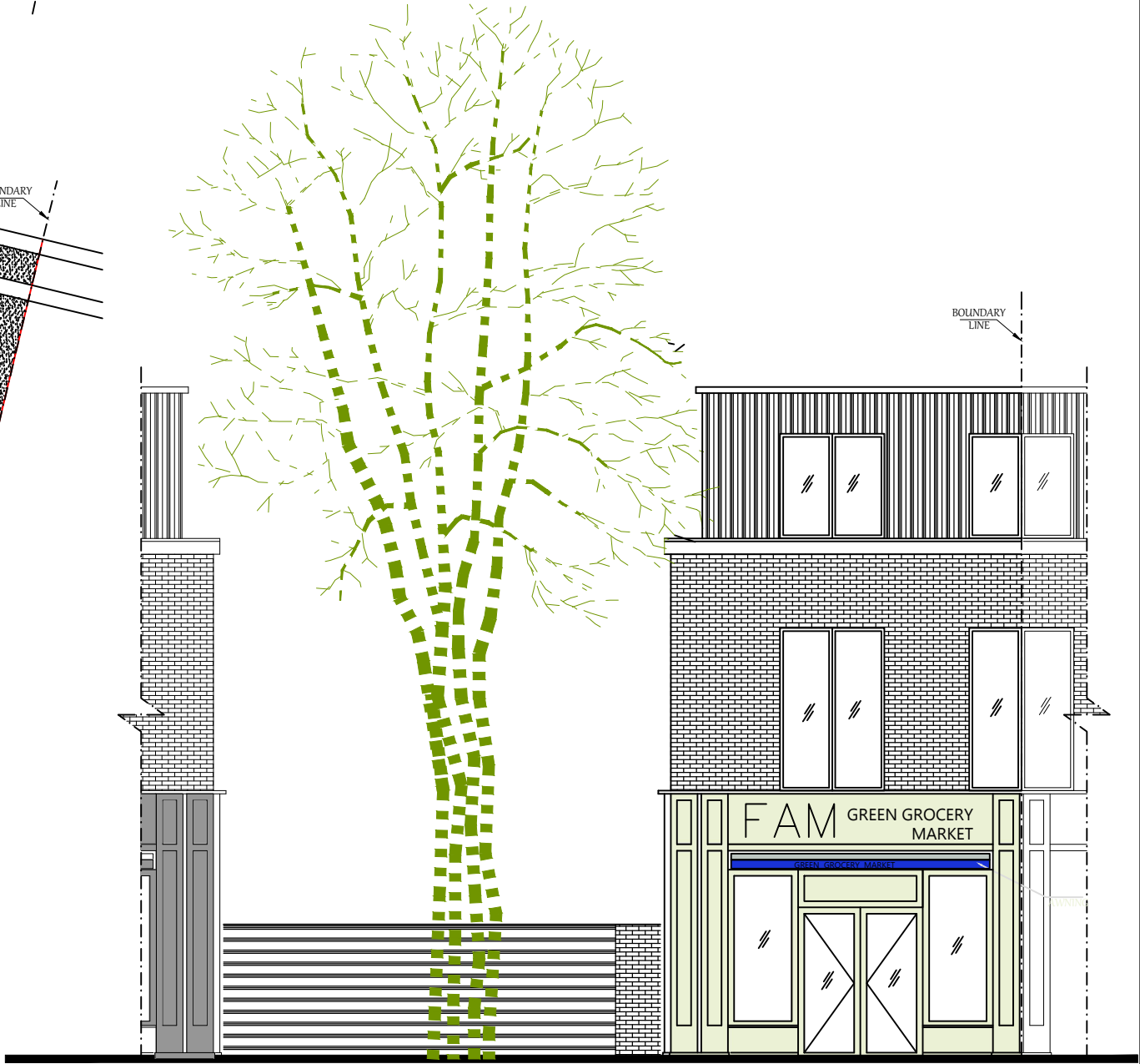
EXISTING FRONT ELEVATION SCALE: 1/100 @A3
