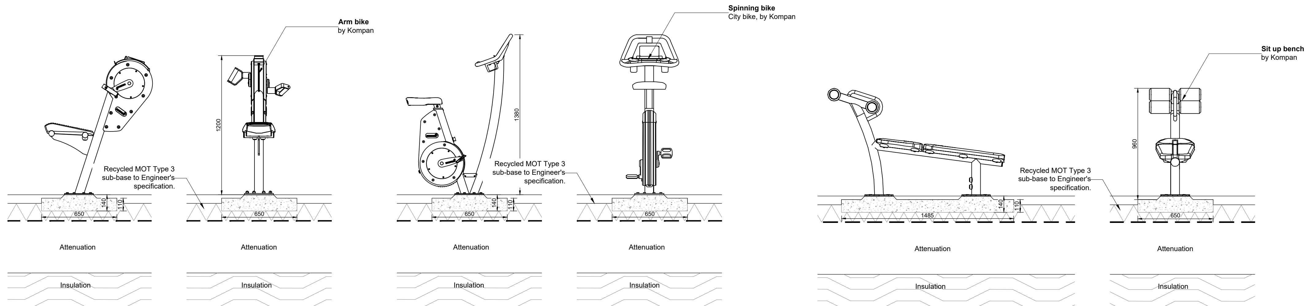
G2 Arm bike Scale: 1:20, Land. spec.: Q52.561
