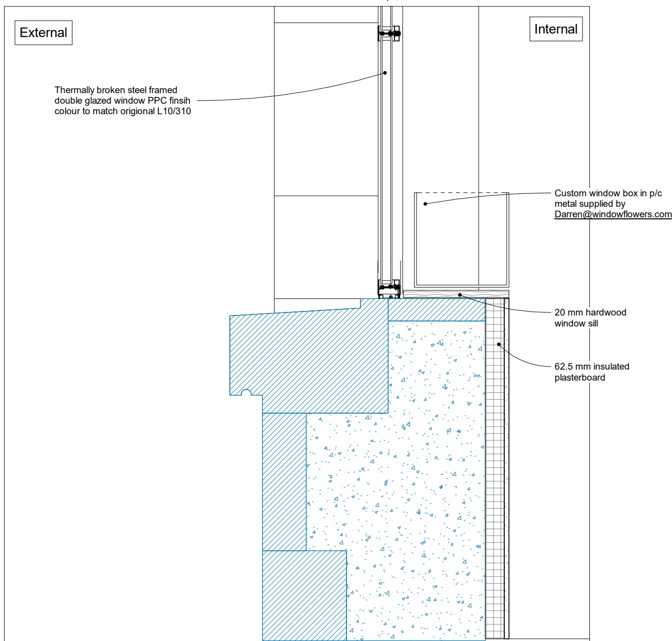
5 W-LG26 Detail Section 1 : 10
