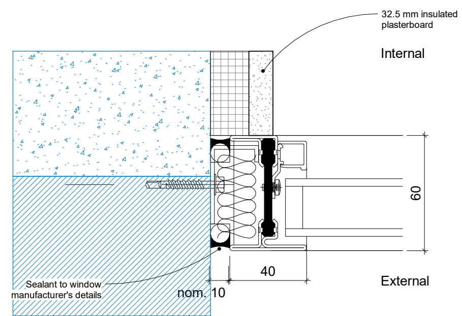
7 W-LG26 Jamn Detail 1 : 2
