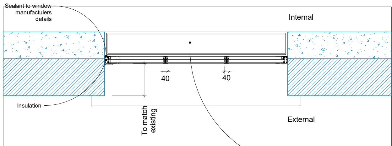
4 W-LG26 Detail Plan 1 : 20
