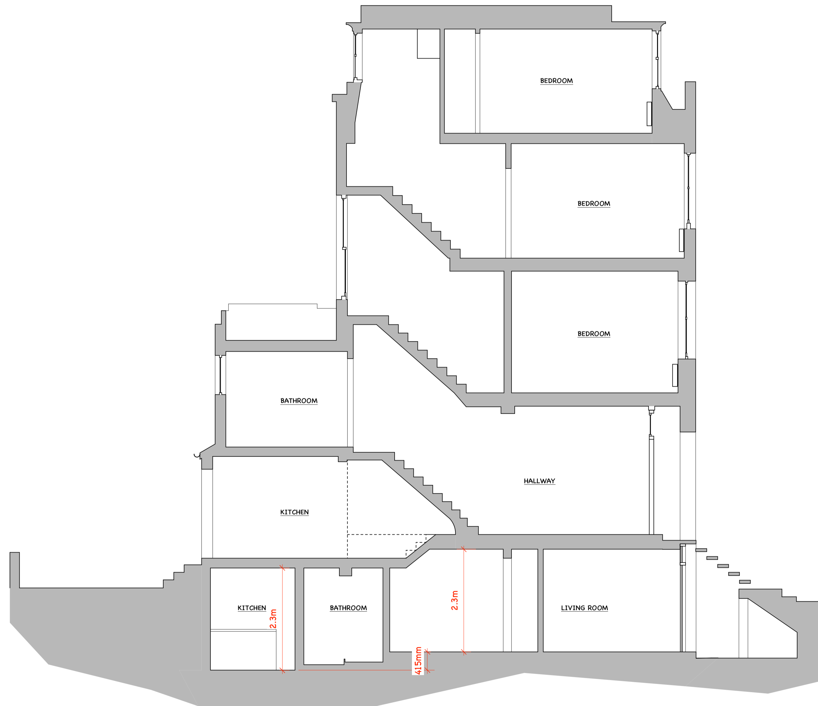
EXISTING SECTION A-A 1:50 @ A1 / 1:100 @ A3
