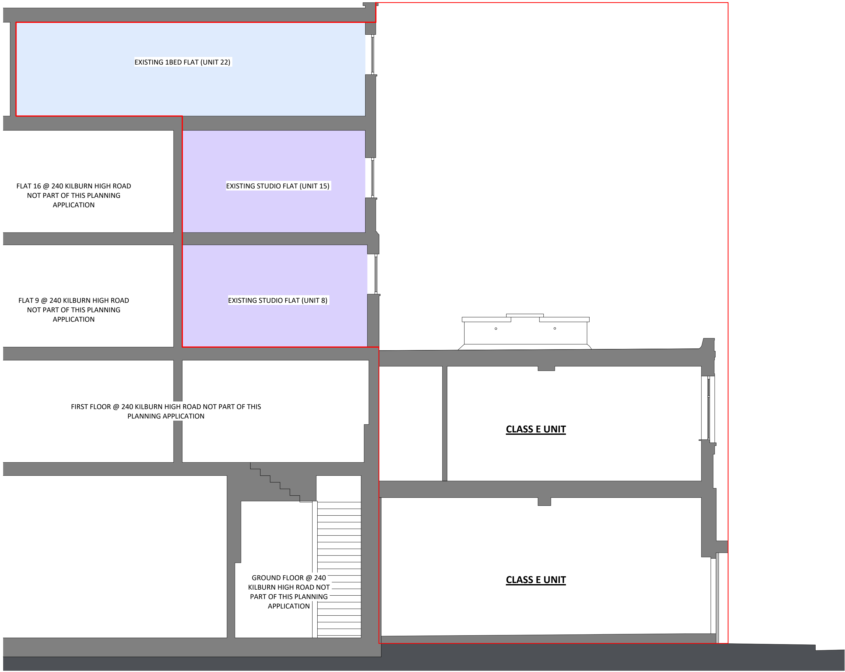
B Existing Section BB 1 : 50 @ A1 / 1:100 @ A3
