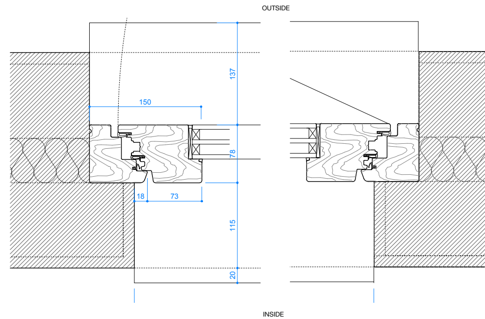
D03_Window Jamb
