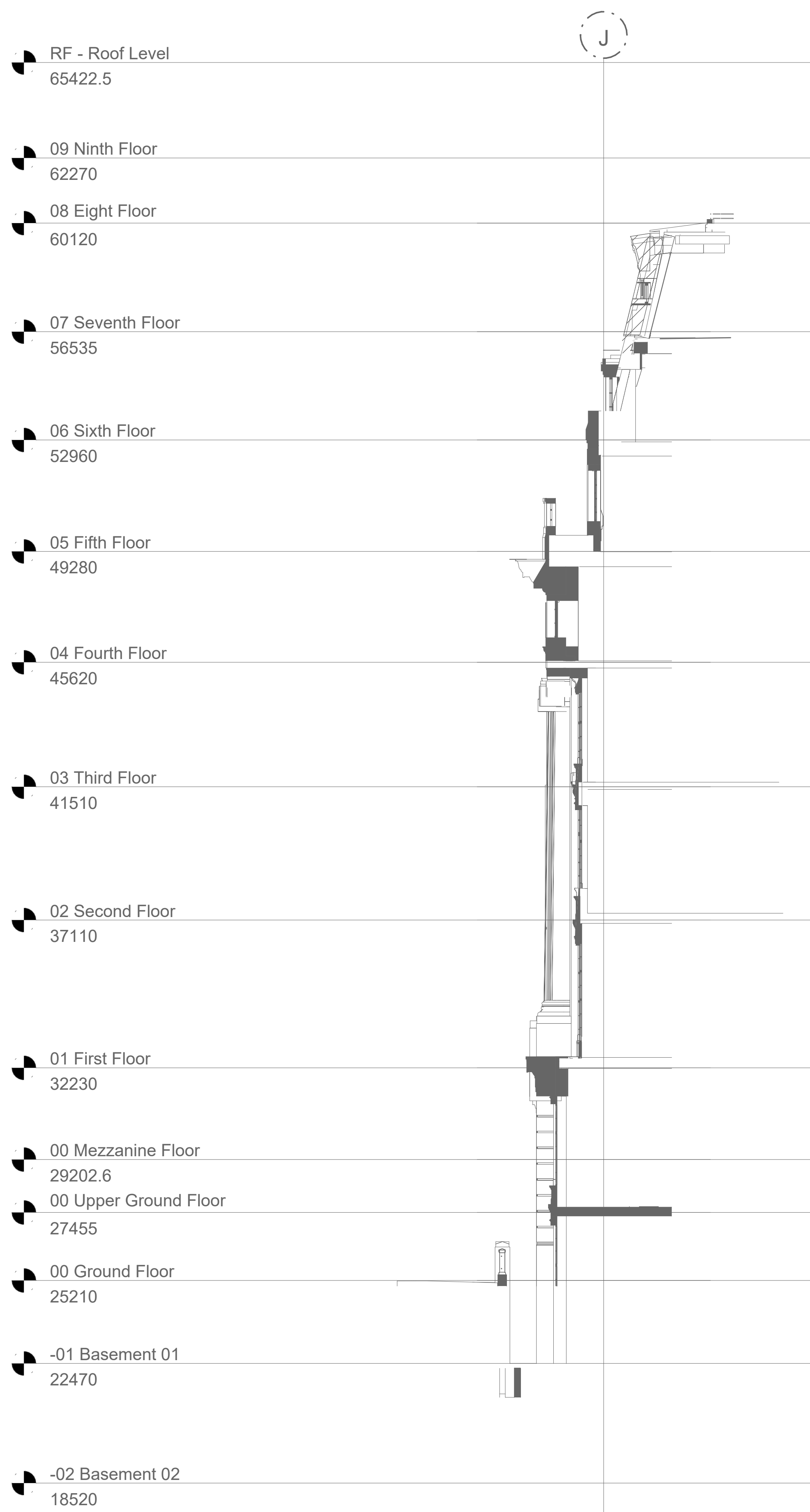
1 Section - Existing - Section A 1 : 100
