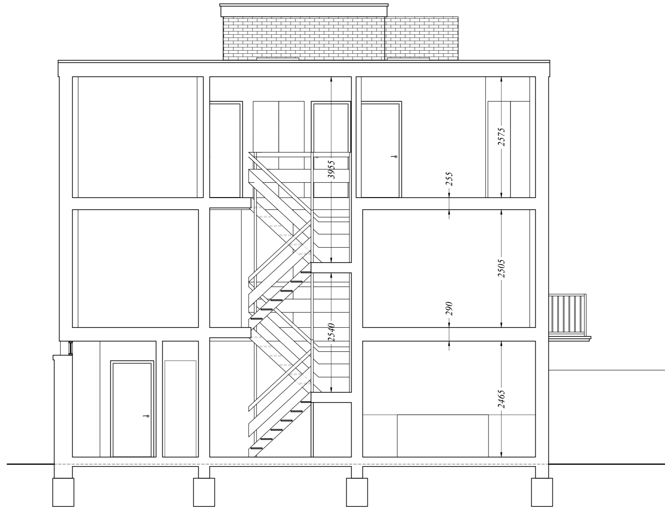
Section A-A
