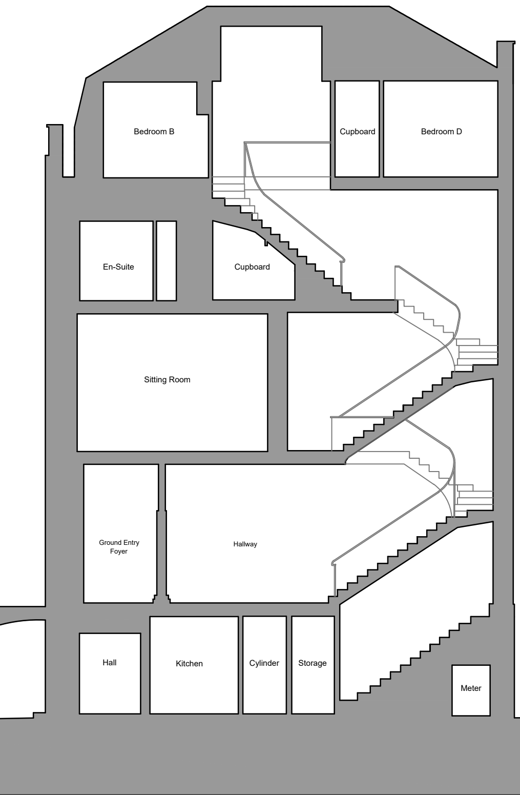
1 Existing Section B-B GHV 1:100 @ A3
