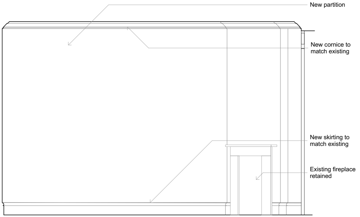
ELEVATION 02
