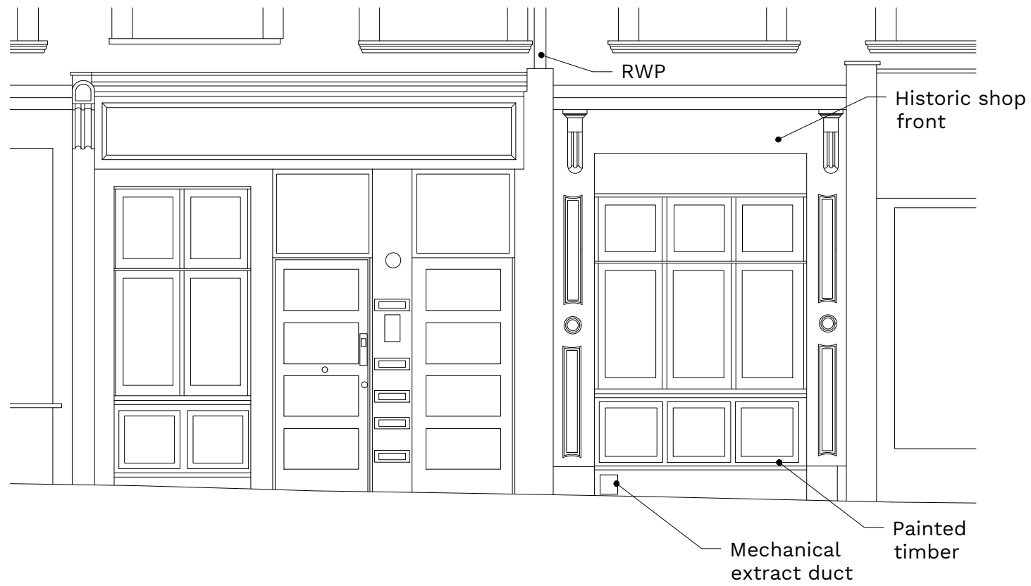
1 EXISTING ELEVATION 1:50 / A3
