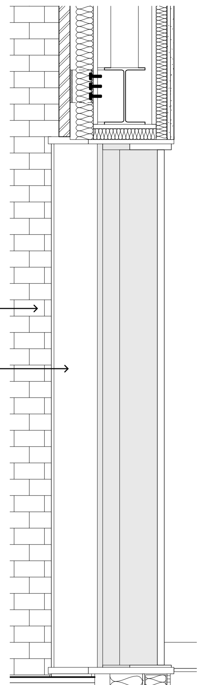
2 Section Scale: 1 : 10
