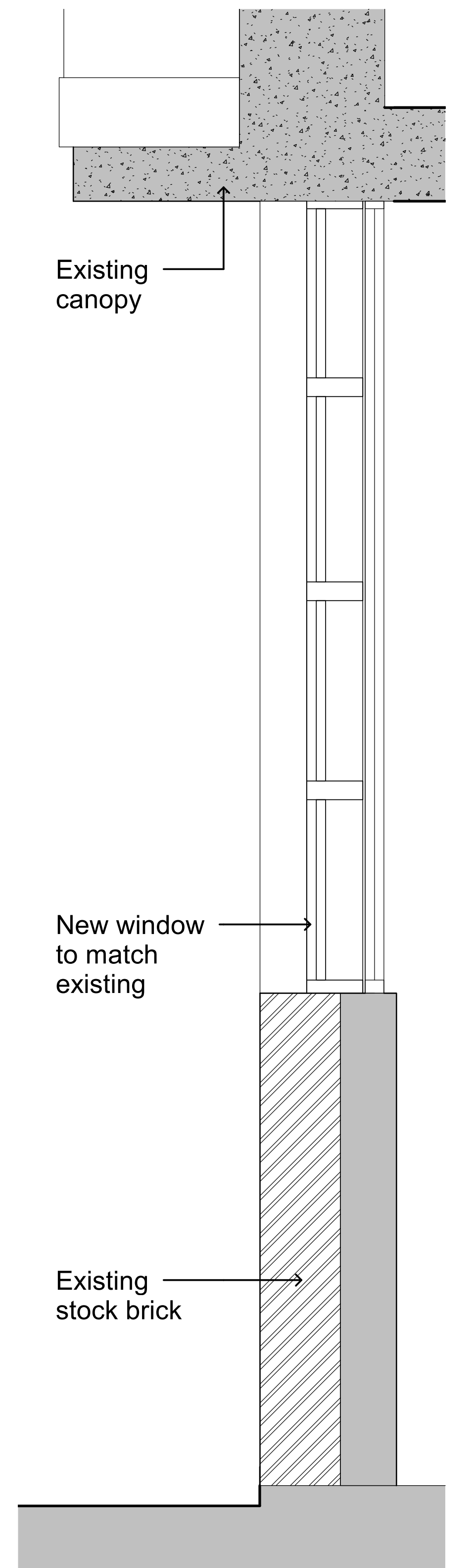
2 Section Scale: 1 : 10
