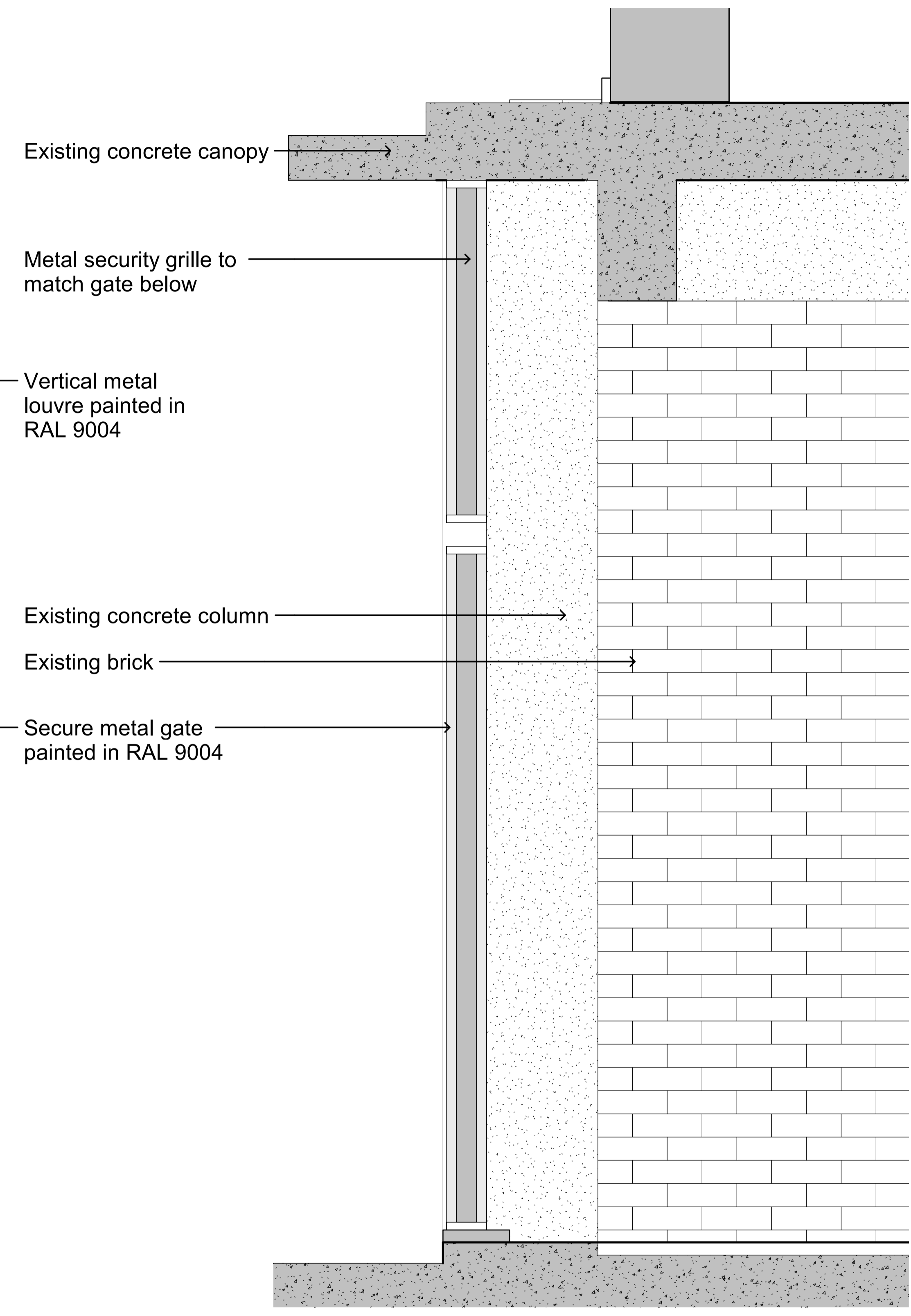
2 Section Scale: 1 : 10
