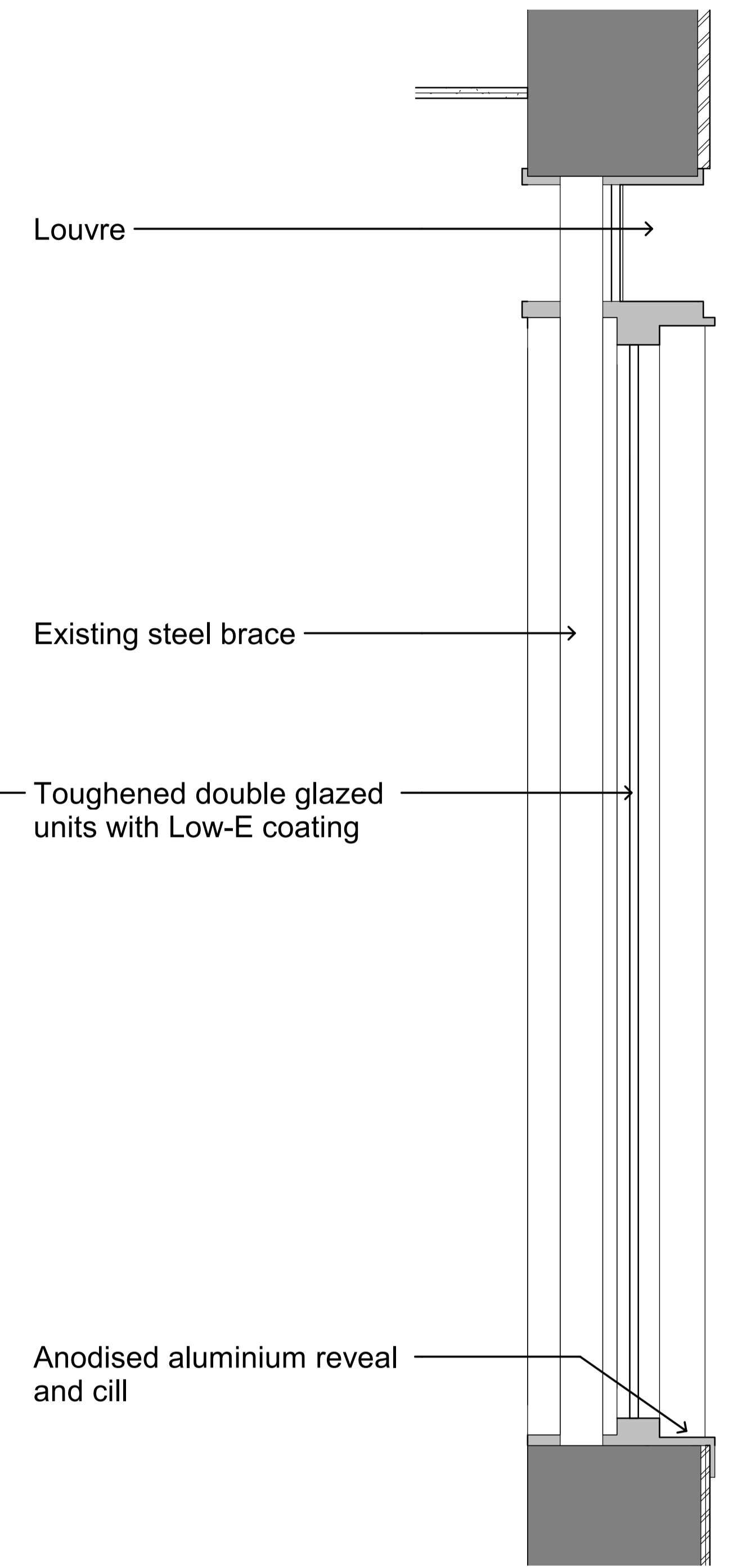
2 Section Scale: 1 : 10
