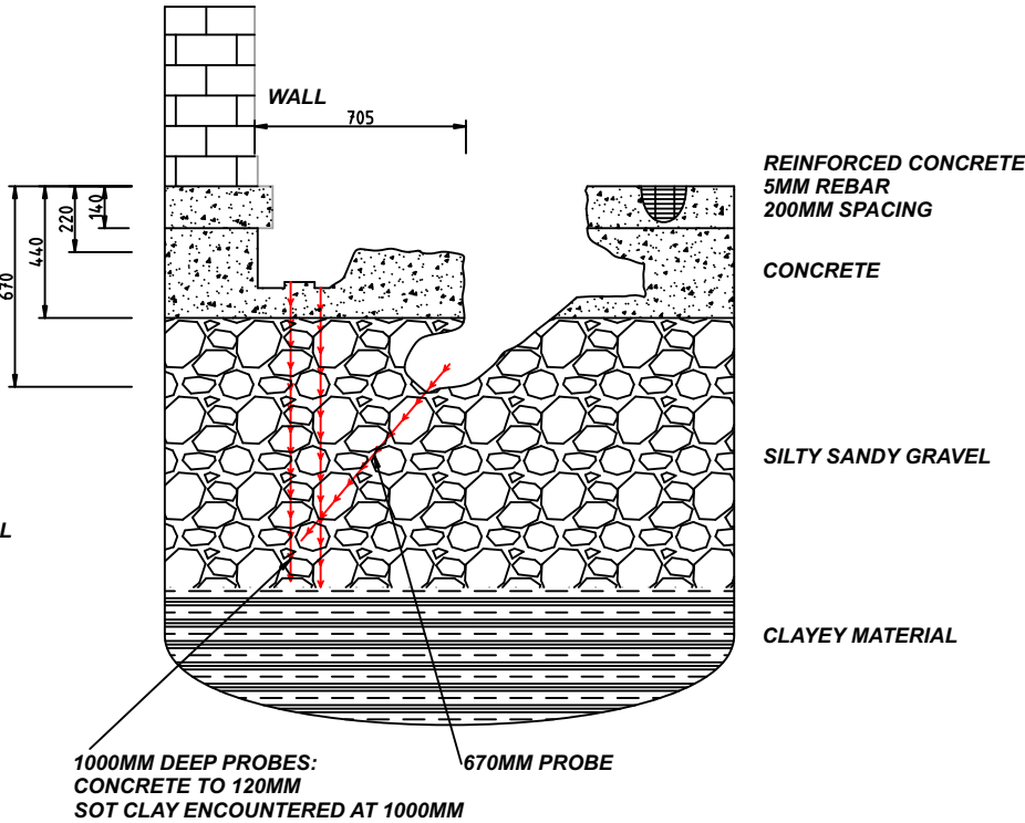
A-A' SECTION
