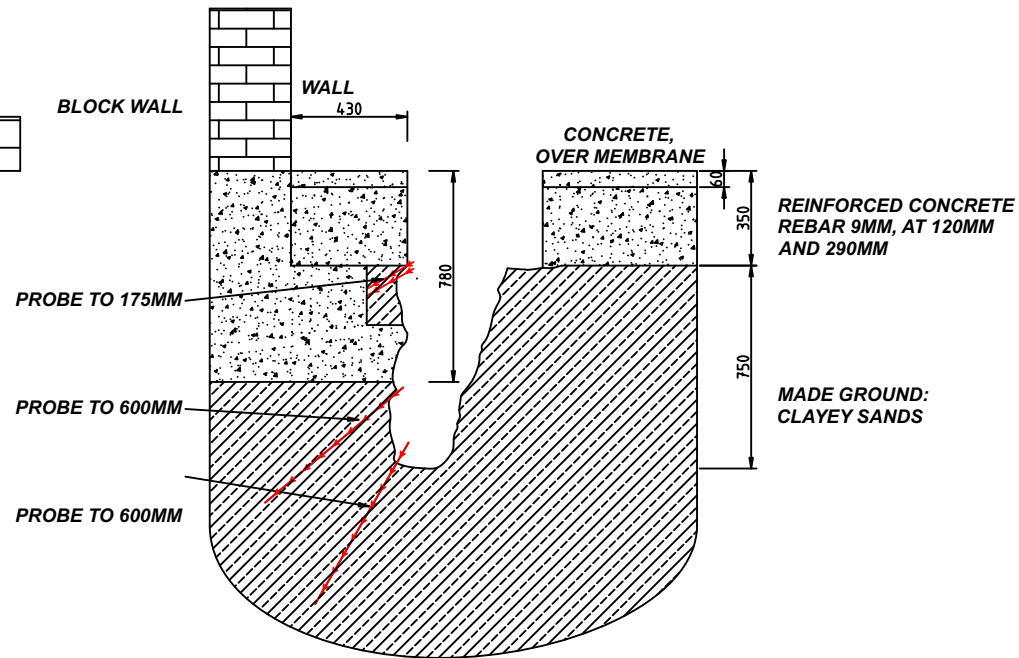
A-A' SECTION
