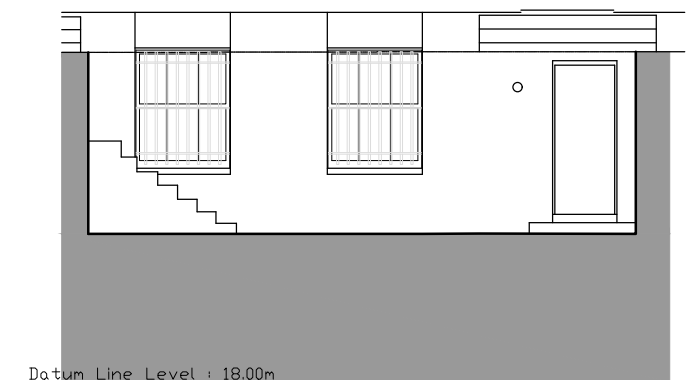
4 Existing Elevation 02 GHV 1:100 @ A3
