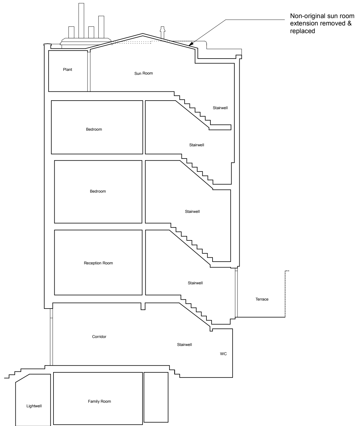
EXISTING SECTION DD
