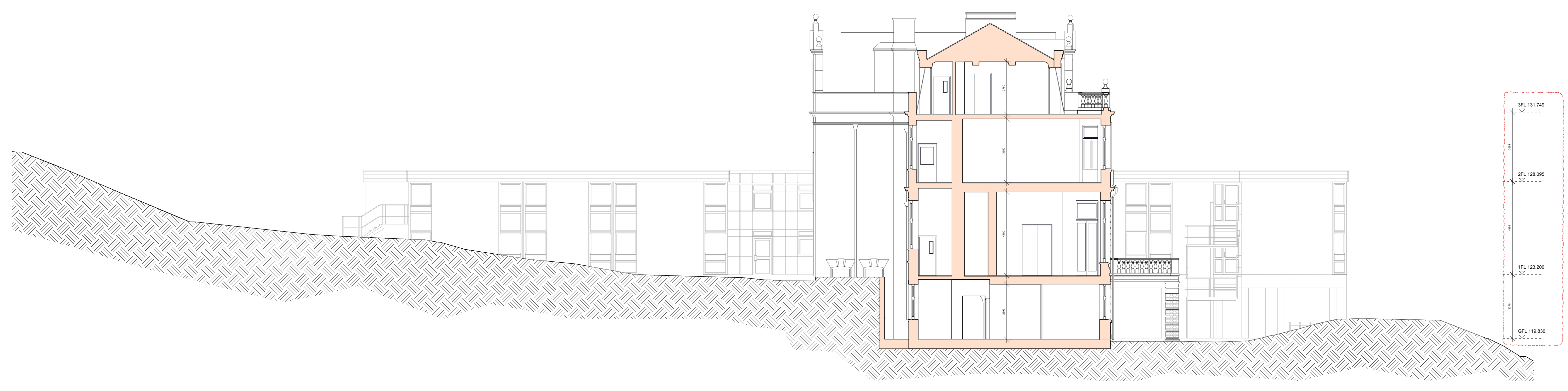
1 EXISTING SECTION A-A PL-09 P01 Scale: 1:100
