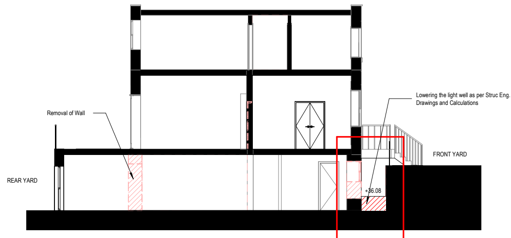
1 Existing Section 1 : 100
