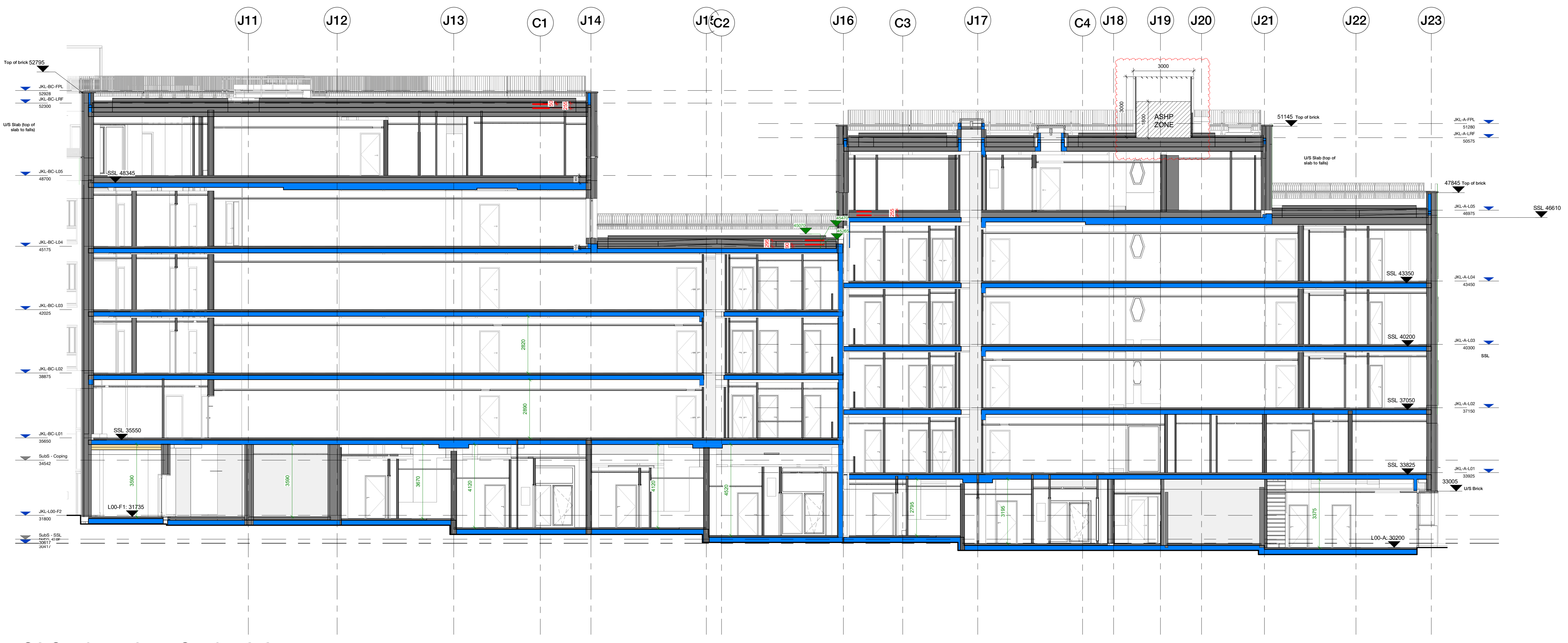
1 GA Sections - Long Section A-A 1 : 100
