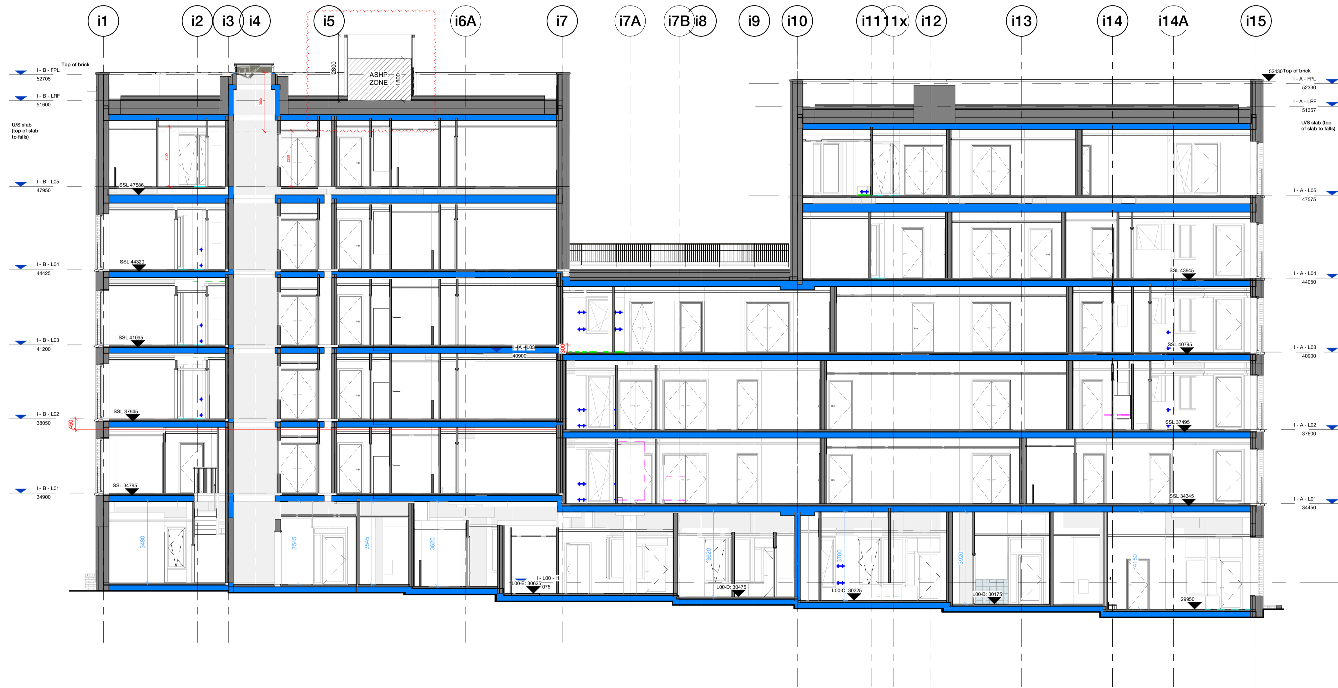
A Long Section A 1 : 100
