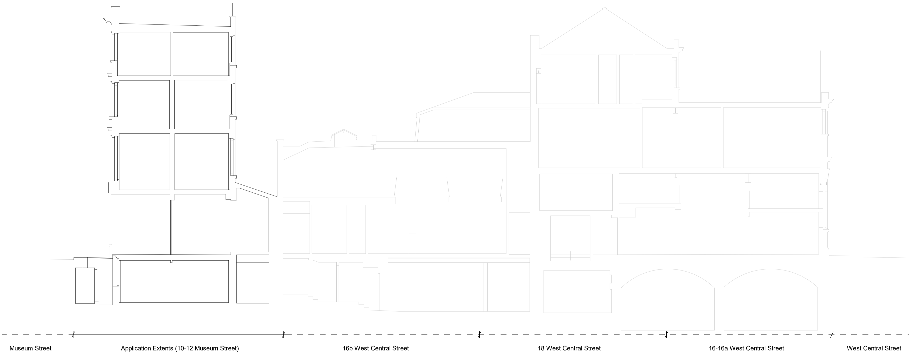
1 WCS - Existing Section BB 1 : 100
