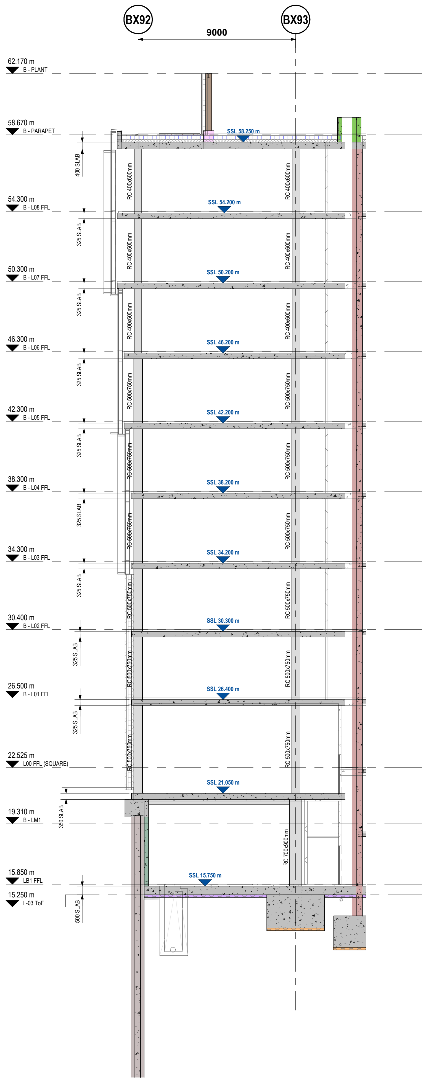
4 Section 4-4 1 : 125
