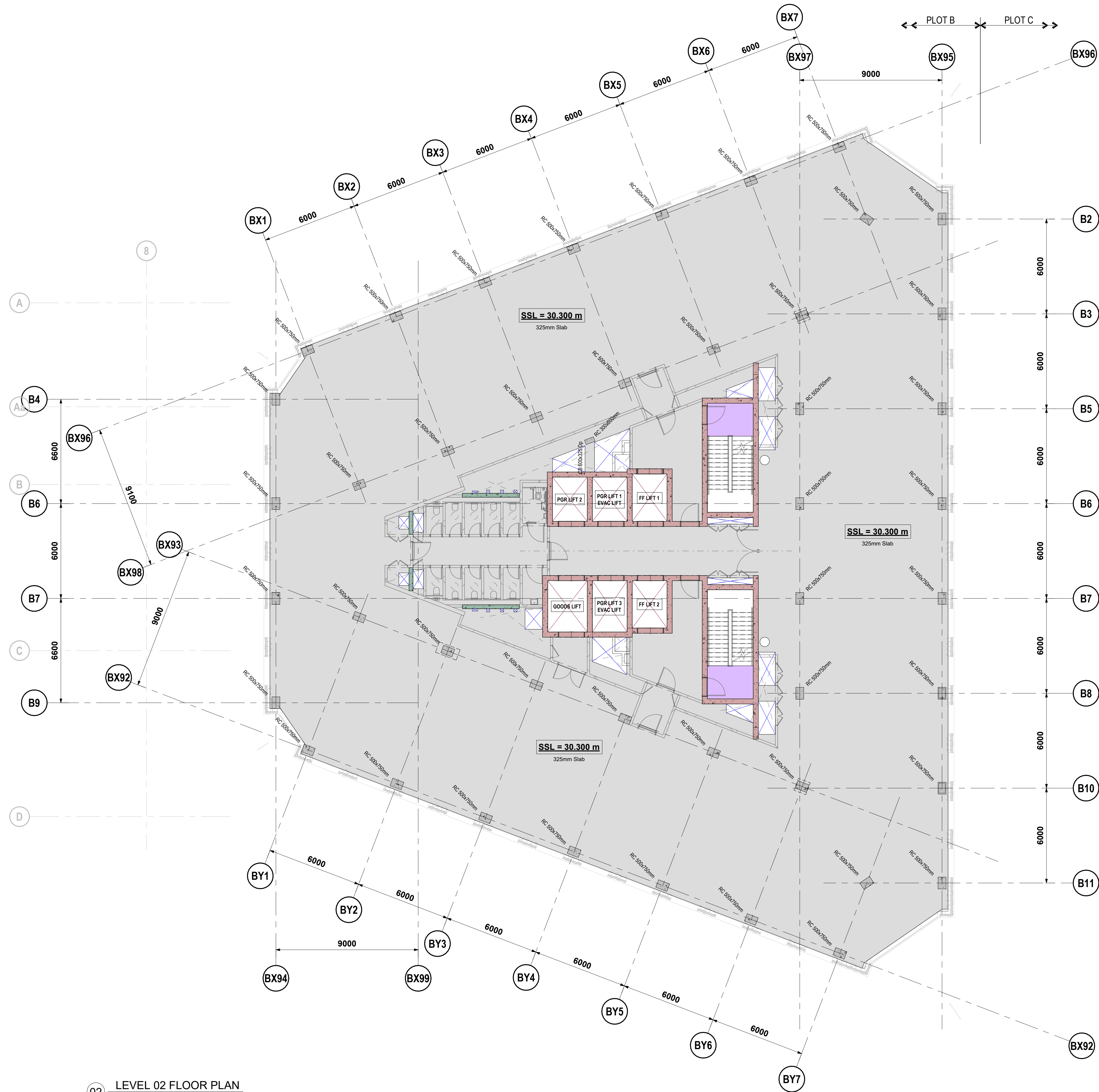
02 LEVEL 02 FLOOR PLAN 1 : 125
