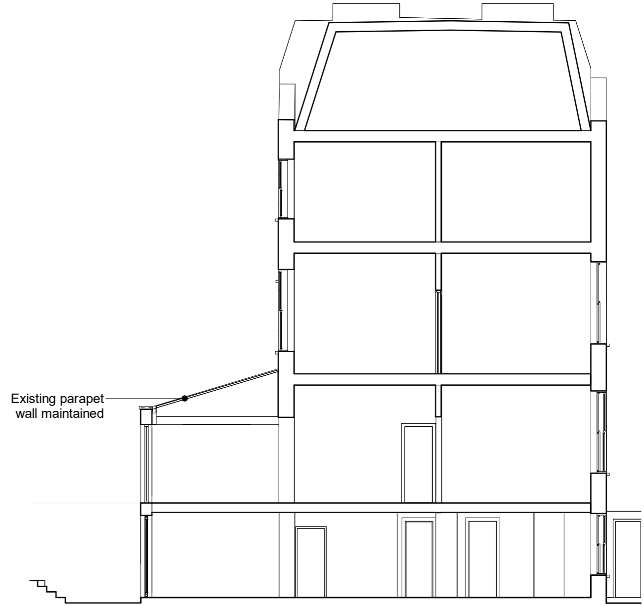
02 Section B-B 1 : 100
