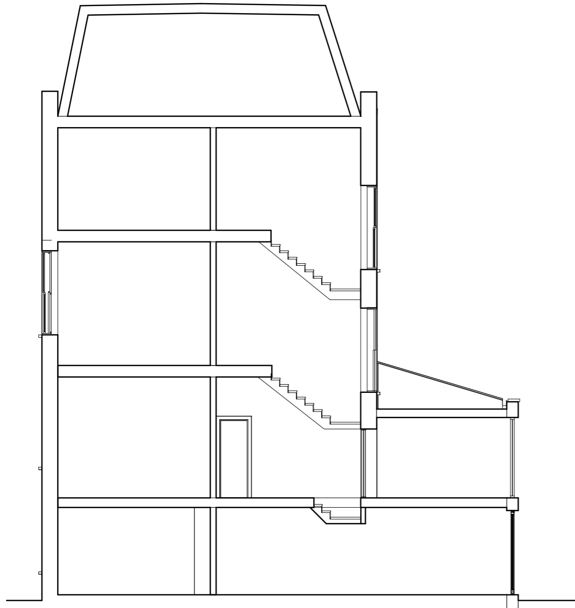
01 Section A-A 1 : 100
