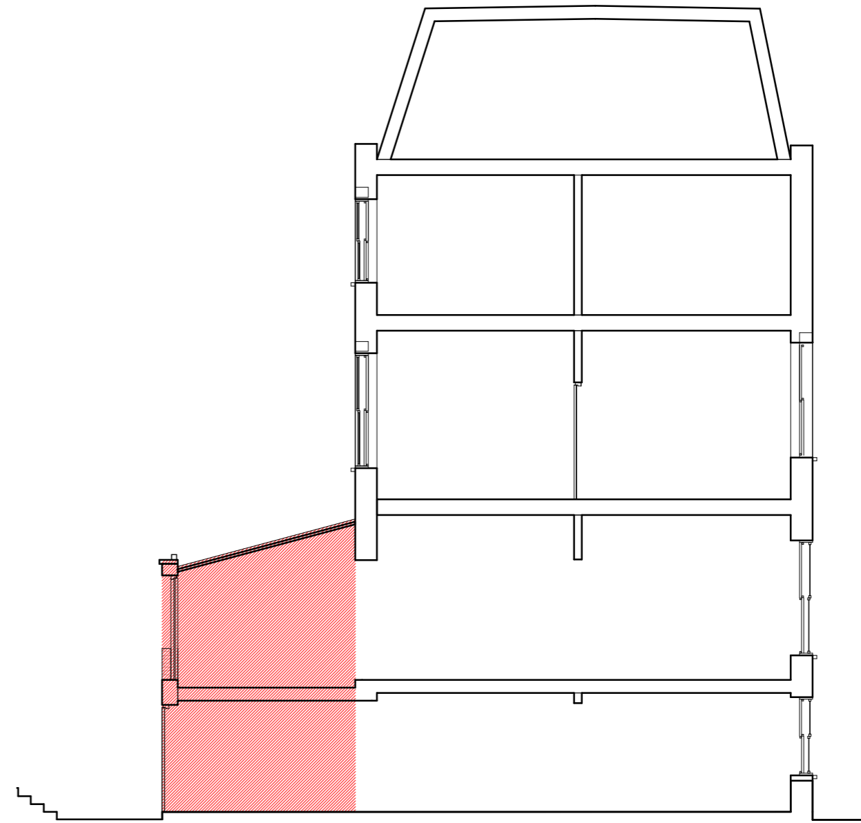
02 Section B-B. 1 : 100
