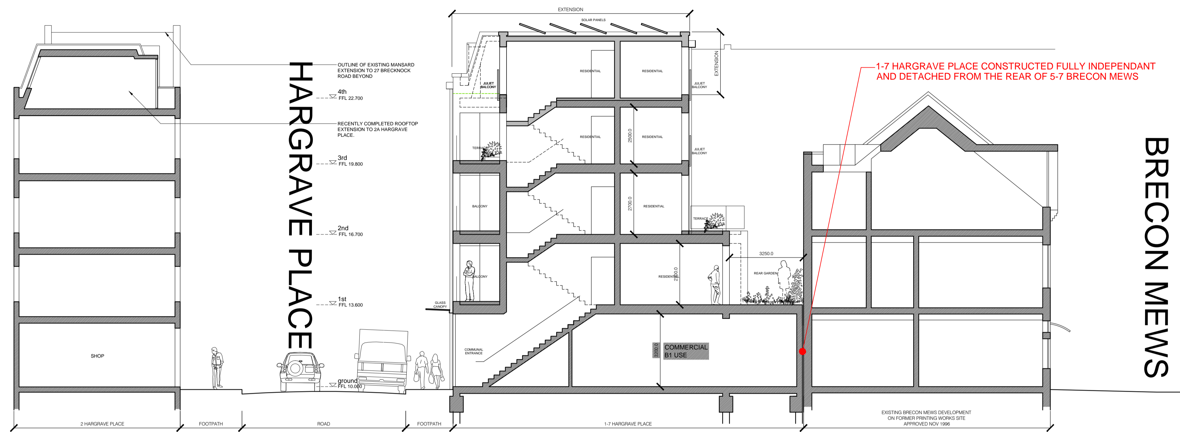
SITE SECTION A-A 1:100 @ A1
