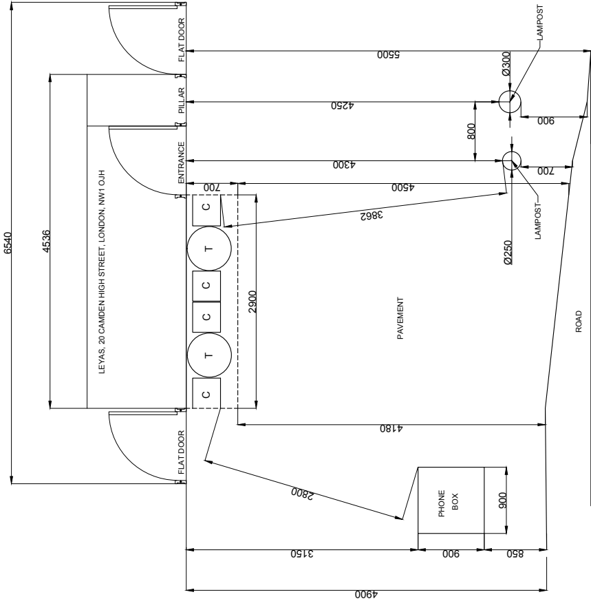
PLAN 1:50
