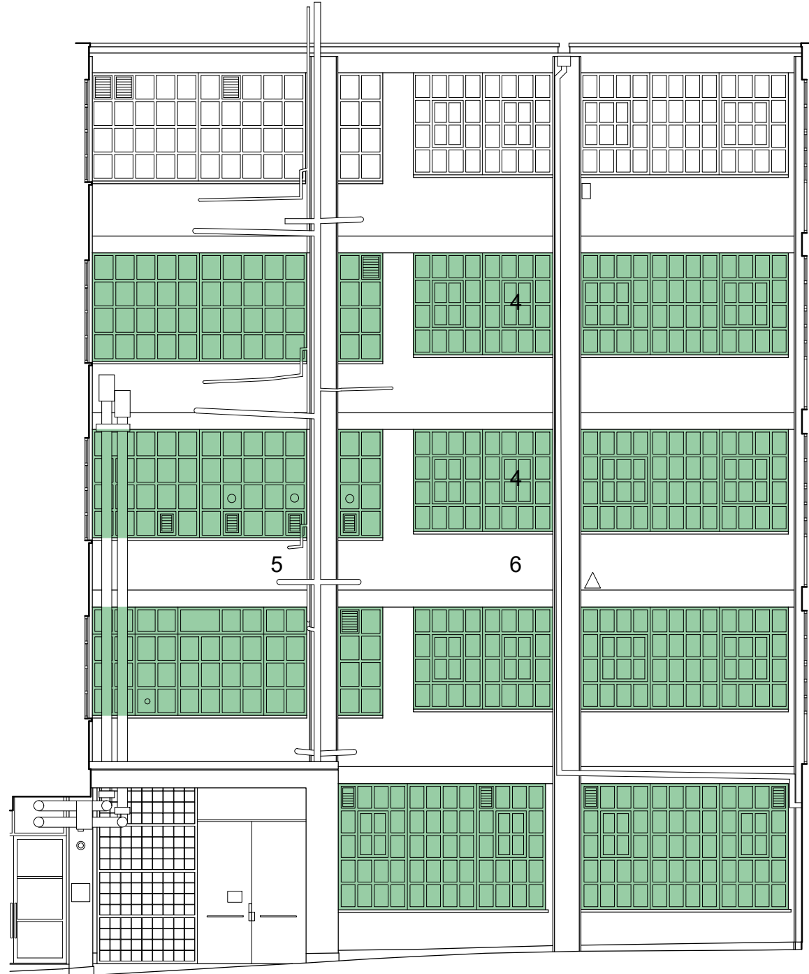
9 Elevation 11
