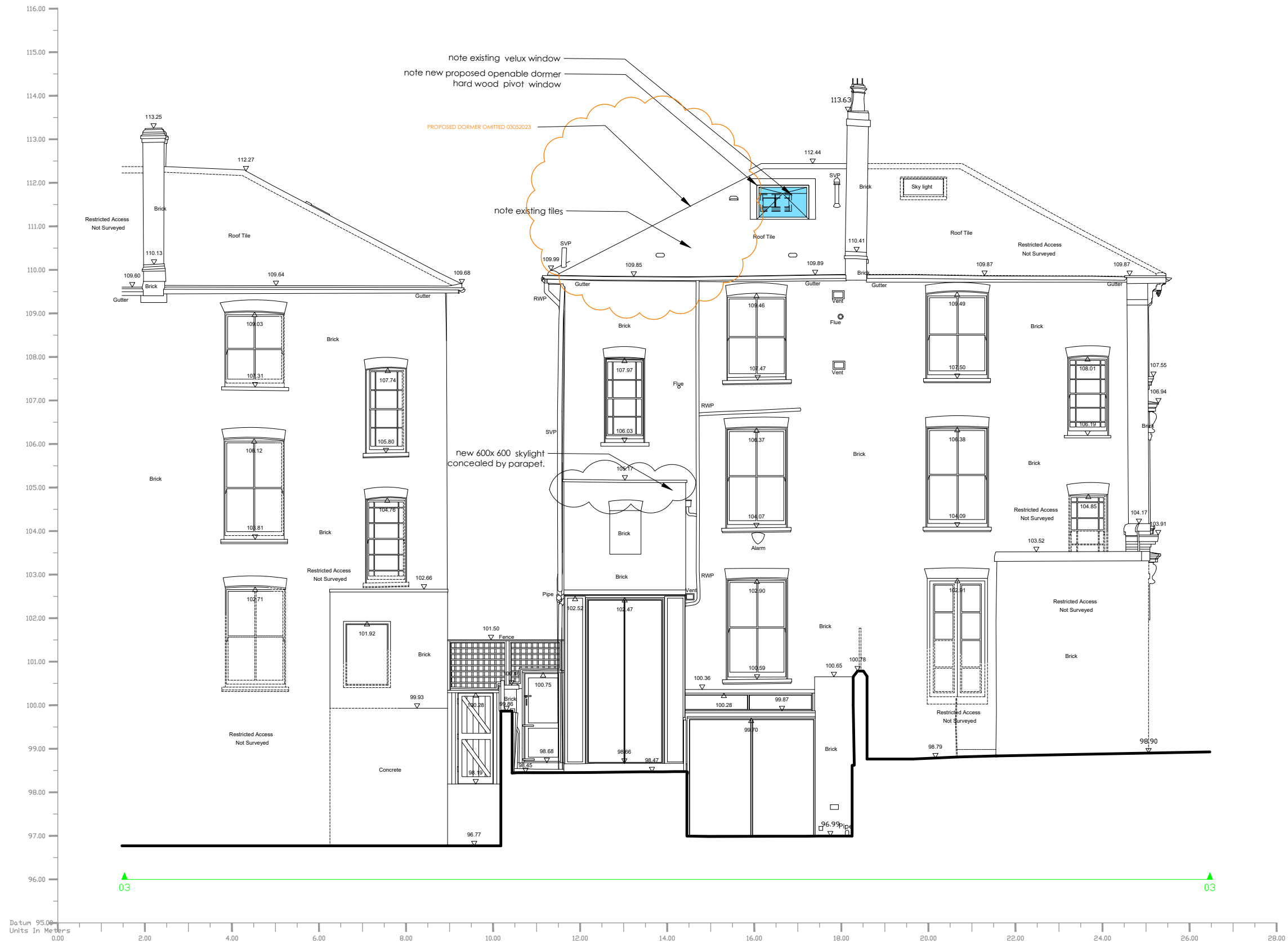
ELEVATION 3
