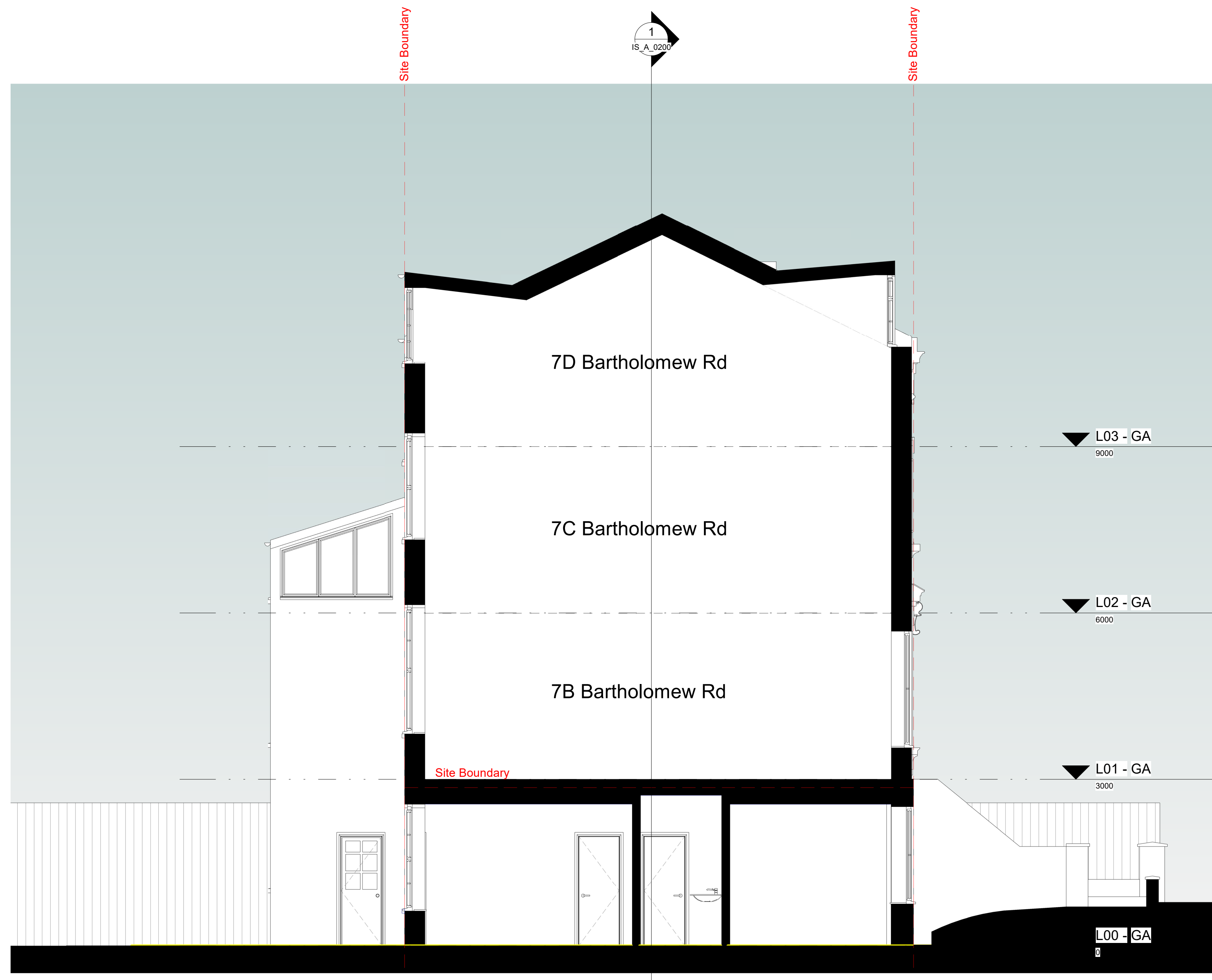
2. Section B-B 1 : 50
