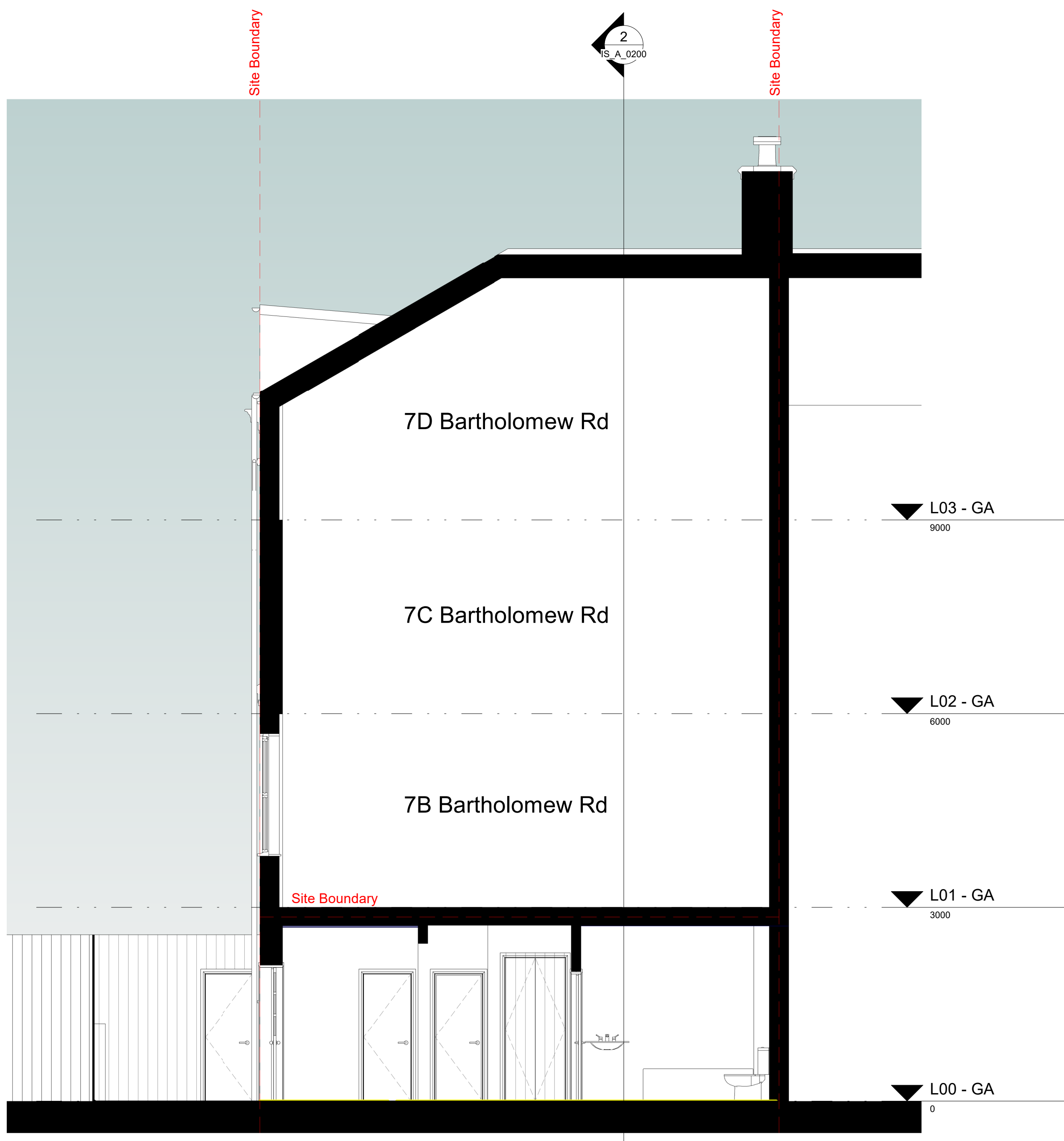
1. Section A-A 1 : 50
