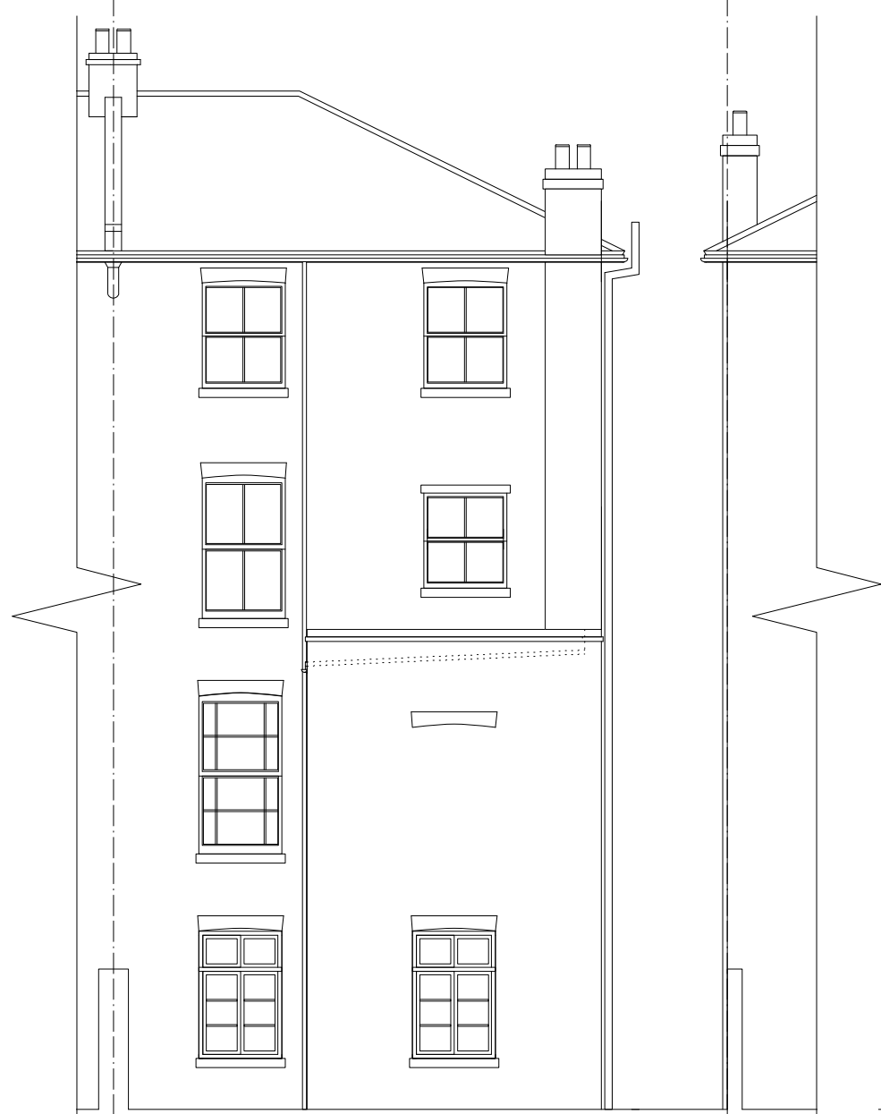
Elevation BB
