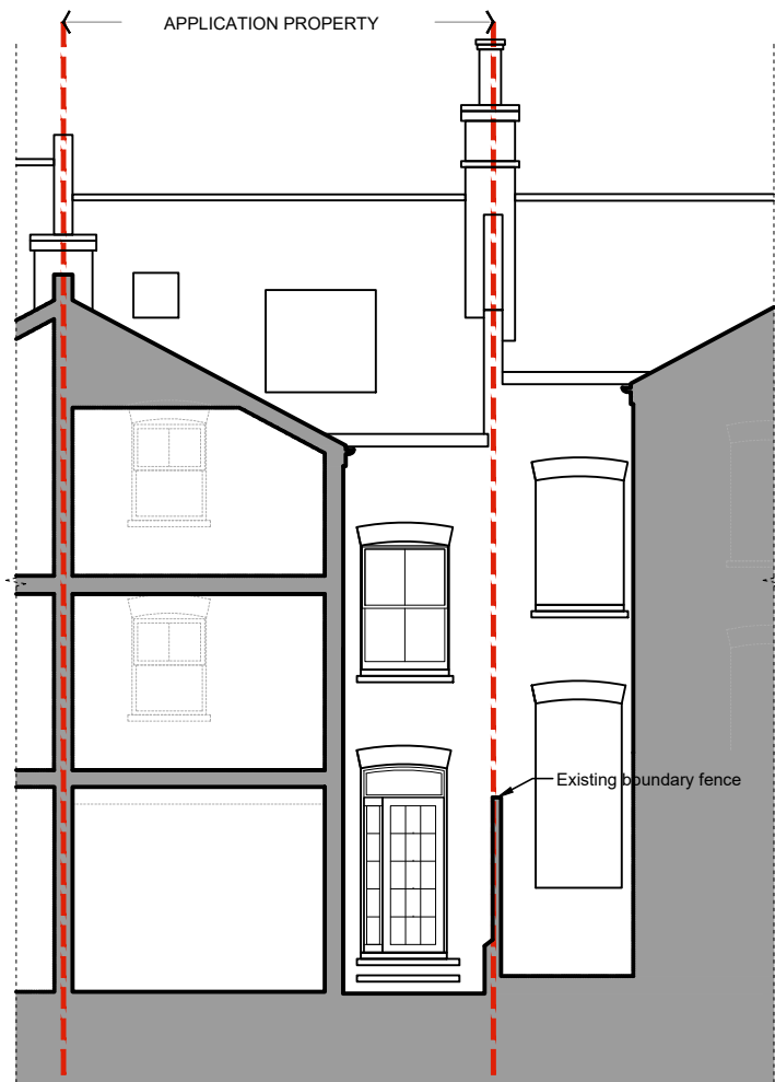
Section A-A
