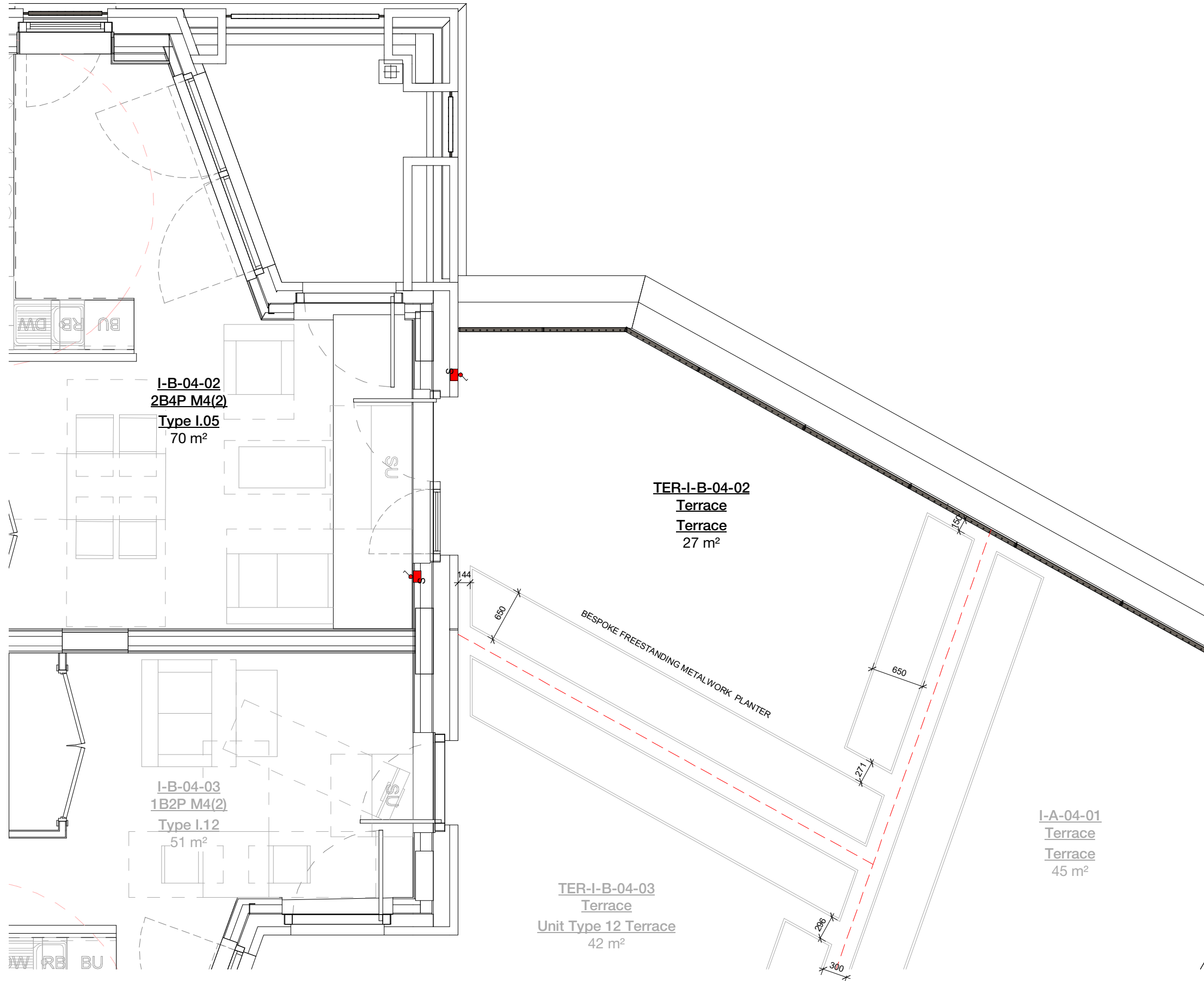
1 Unit Type 5 Terrace Plan 1 : 50
